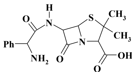
Ампіцилін
