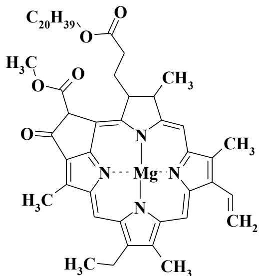
Хлорофіл-α
