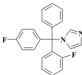
Флутримазол
