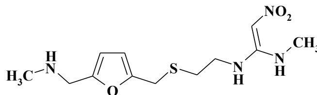
Ранітидин
