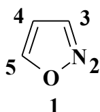
Ізооксазол
