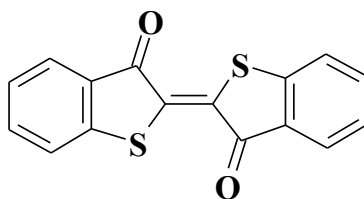
Тіоіндиго
