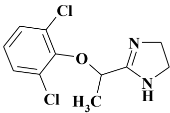
Лофексидін
