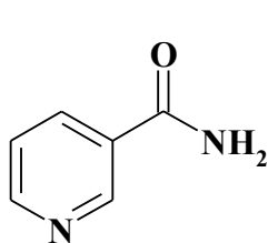
Нікотинамід
