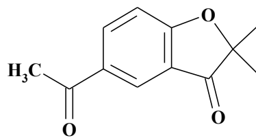
Спізофурон
