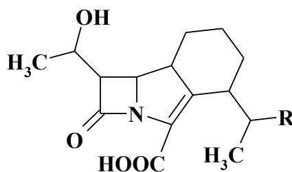
Тринеми
