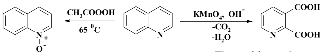
N-Оксид хіноліну
