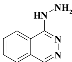
Гідралазін
