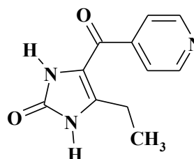
Піроксімол
