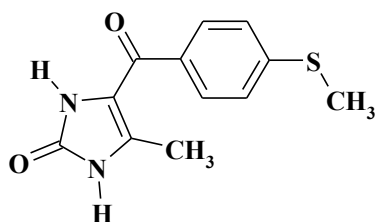
Еноксімол
