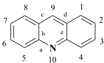
Акридин
