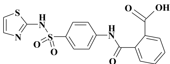
Фталазол
