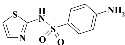
Норсульфазол
