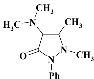
Амідопірін
