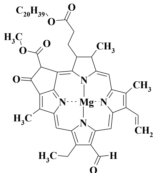
Хлорофіл-β
