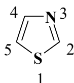
Тіазол
