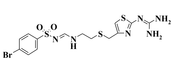
Ебротидин
