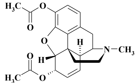
Героїн
