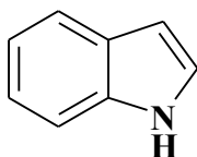
Індол
