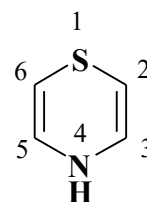
4H-1,4-Тіазин
