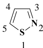
Ізотіазол
