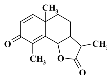
Сантонін
