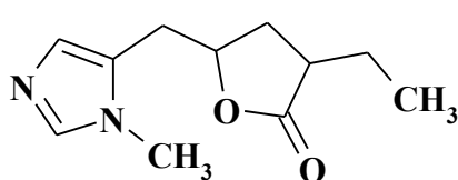
Пілокарпін
