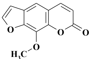
8-Метоксипсорален
