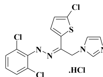
Зіноконазол
