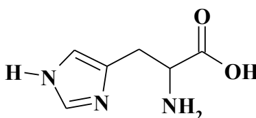
Гістидин
