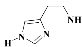
Гістамін
