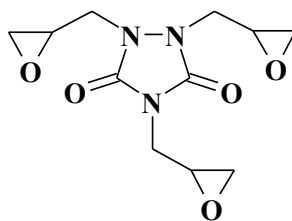
Анаксирон
