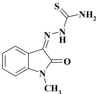
Тіосемикарбазон 1-метилізатину
