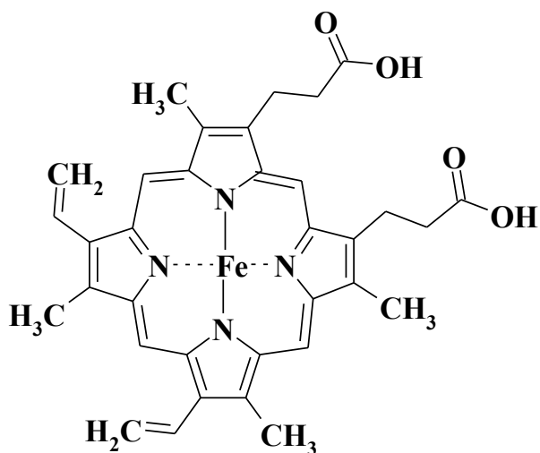
Гем
