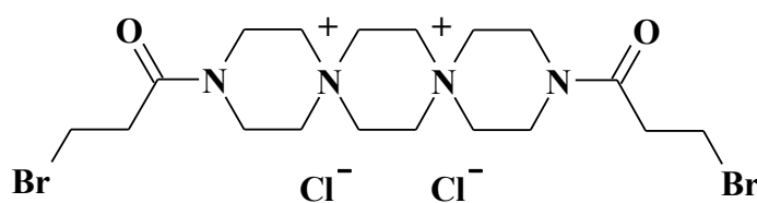
Спіробромін
