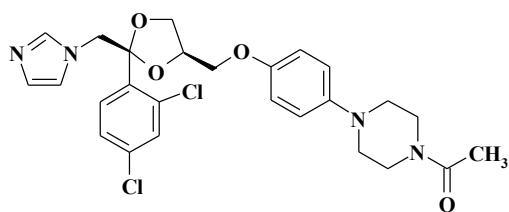
Кетоконазол
