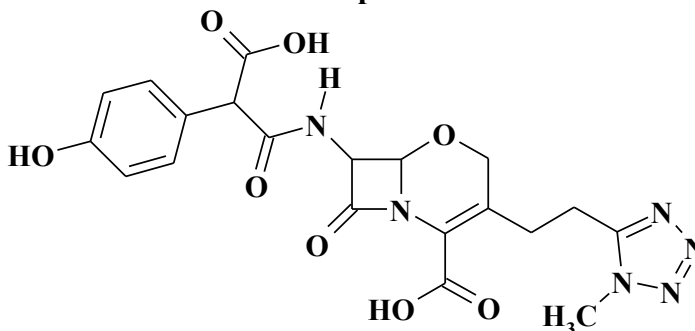
Моксілактам
