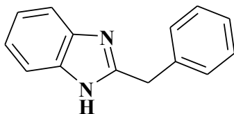
Дібазол
