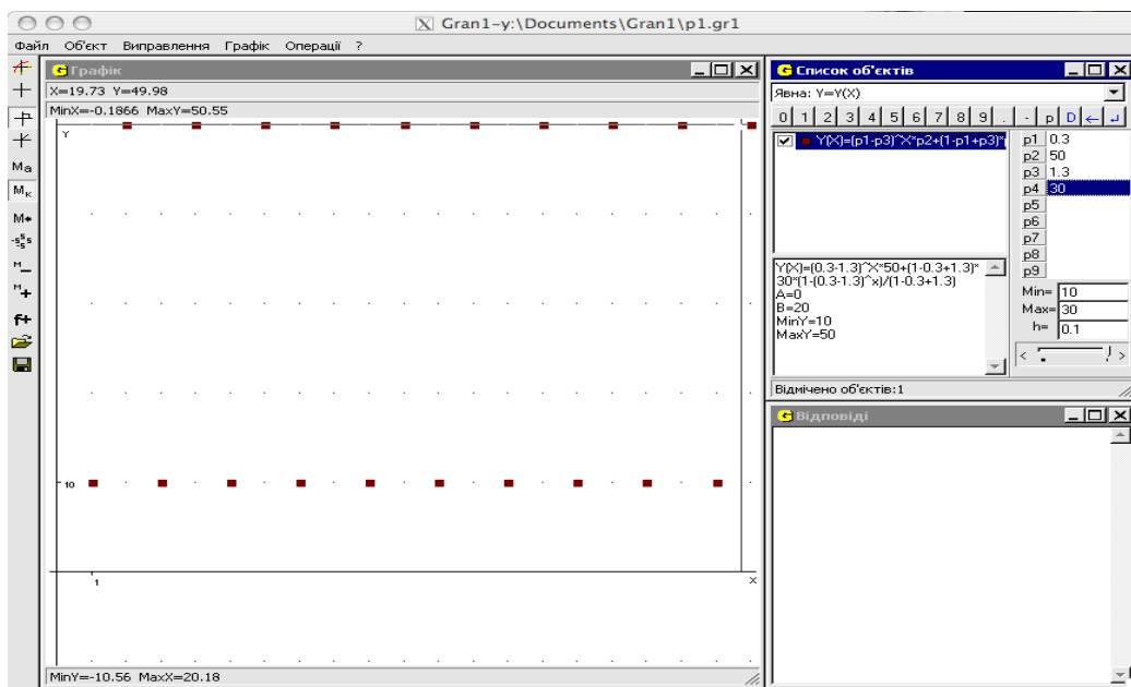
Рис. 4.33. Чисельність популяції по черзі набуває двох значень.
