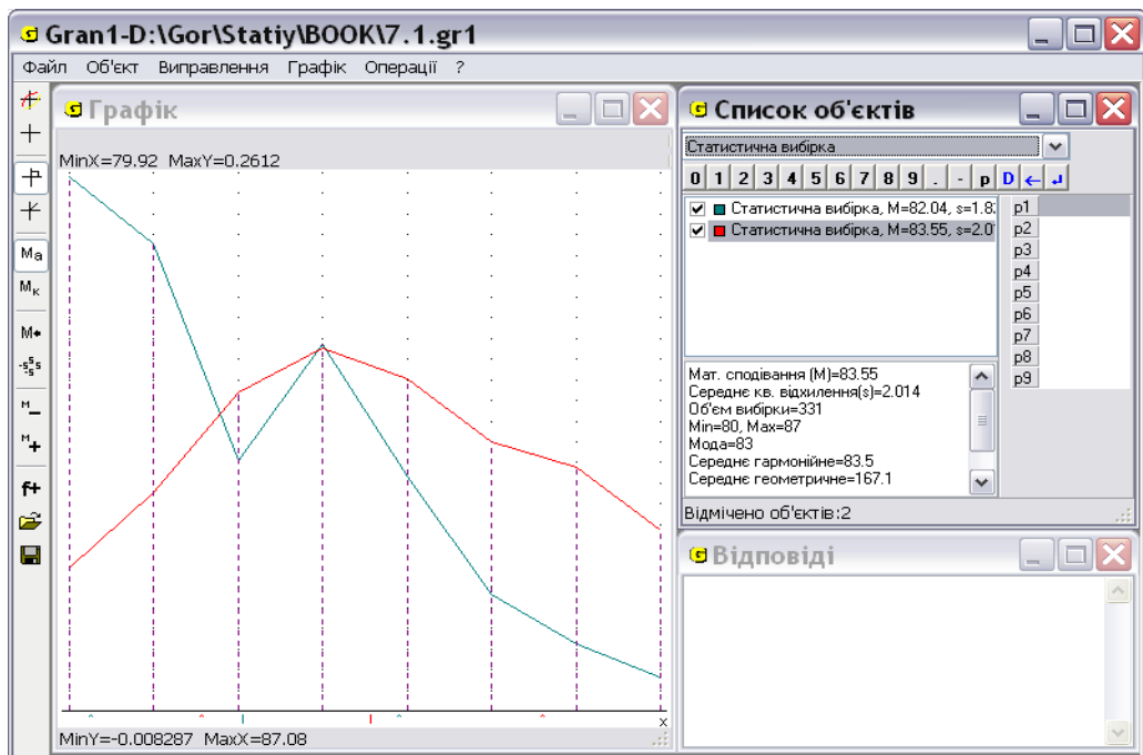
Рис. 4.8. Полігони відносних частот до Задачі 4.14.
