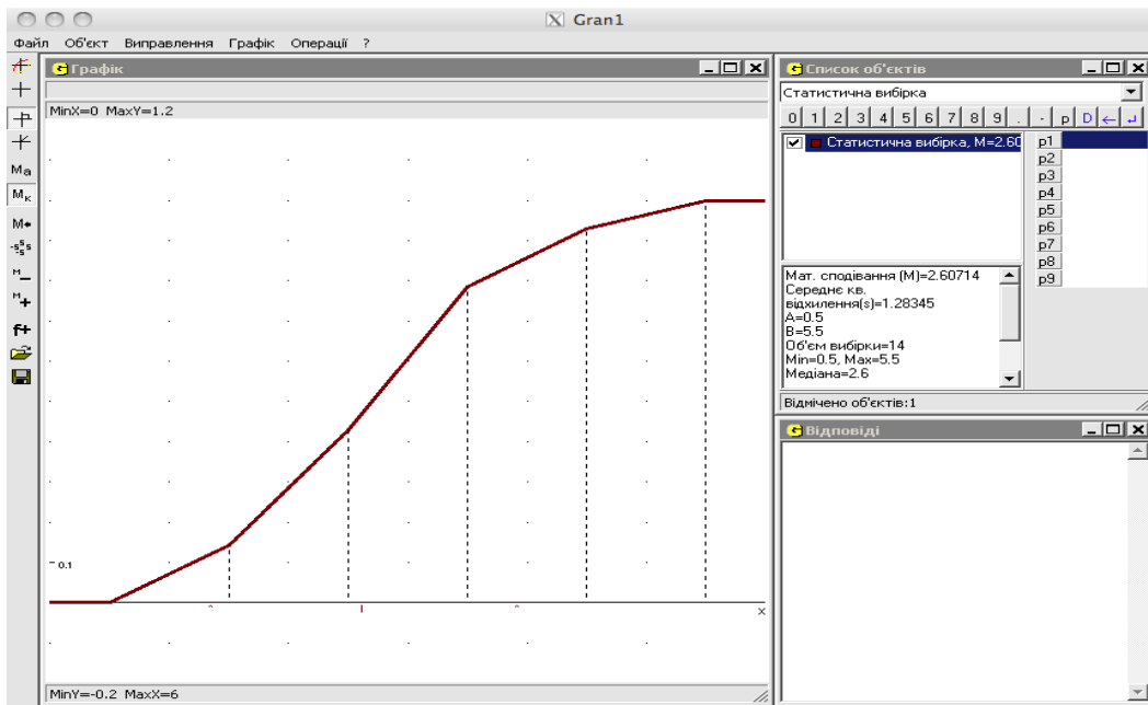
Рис. 2.30. Функція неперервного розподілу статистичних ймовірностей.
