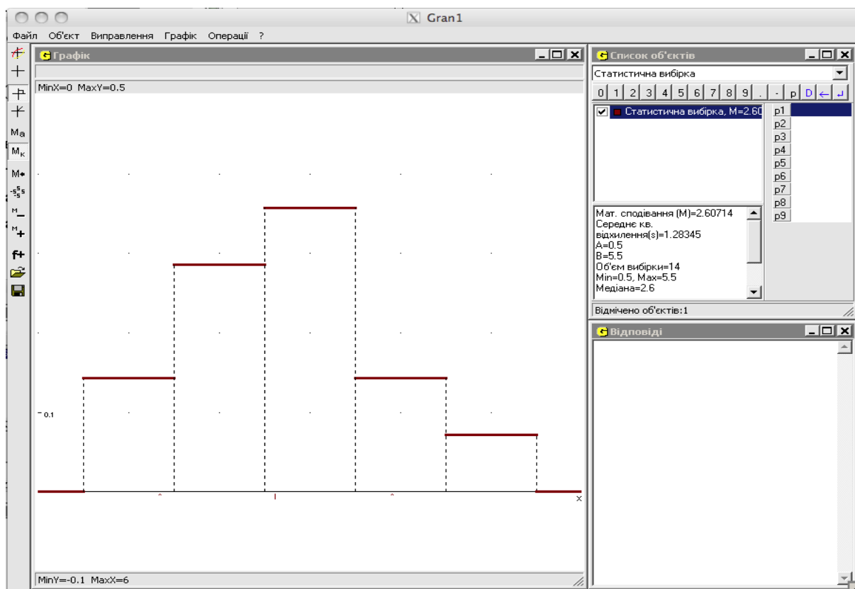
Рис. 2.27. Гістограма.
