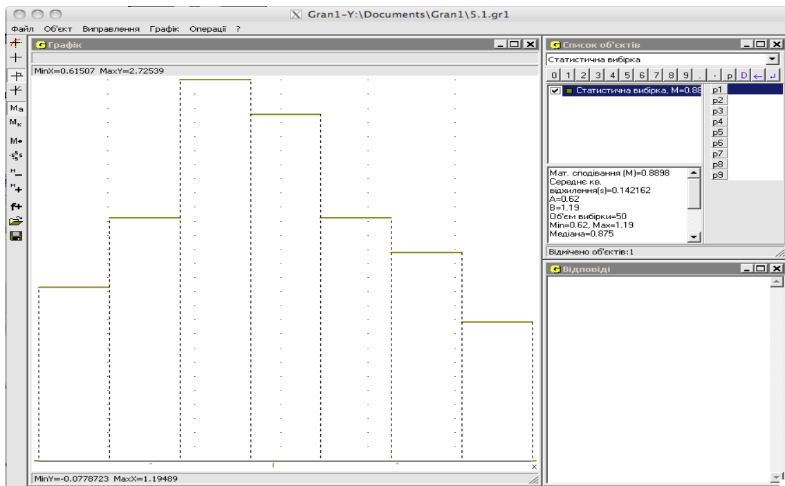
Рис. 4.9. Гістограма до Задачі 4.3.
