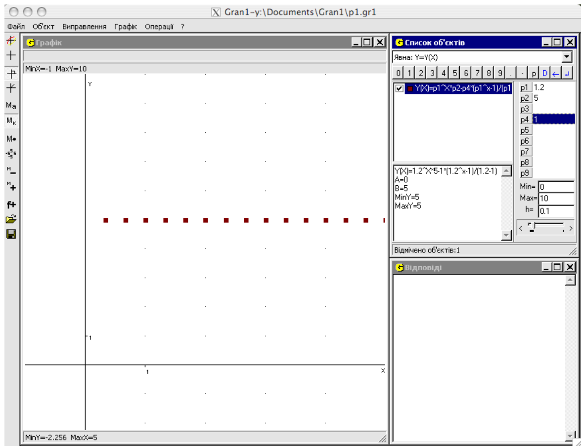
Рис. 4.30. Графік стабільної чисельної популяції.
