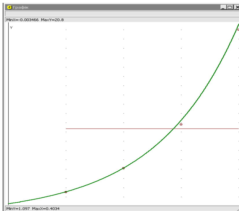
Рис. 4.25. Графік функції до Задачі 4.39.
