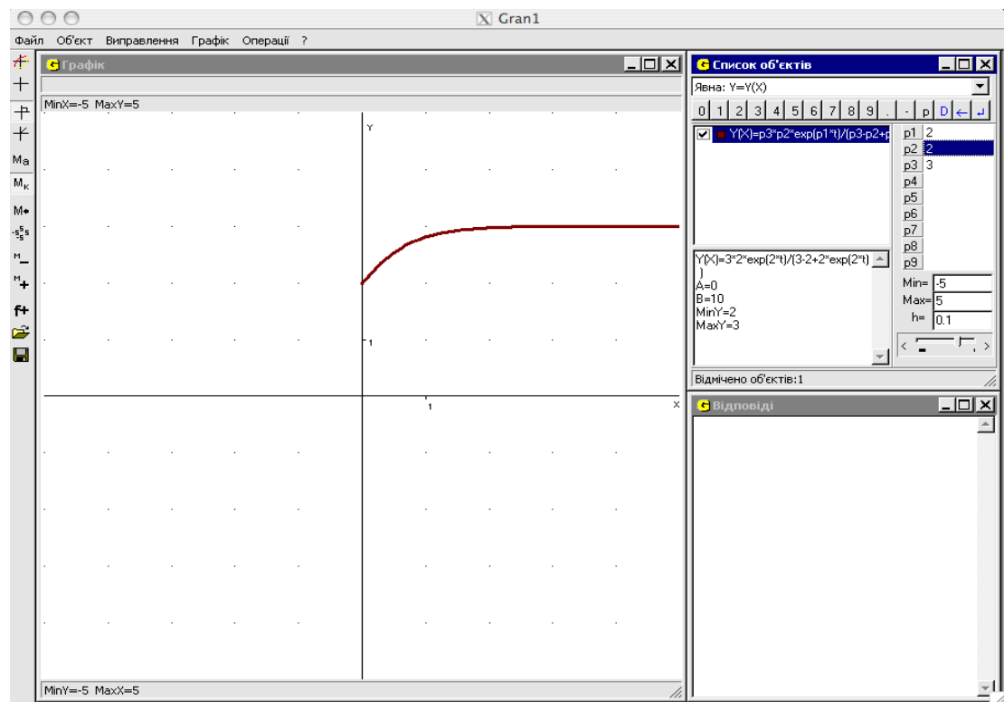
Рис. 4.37. Чисельність популяції зростає до демографічної ніші.
