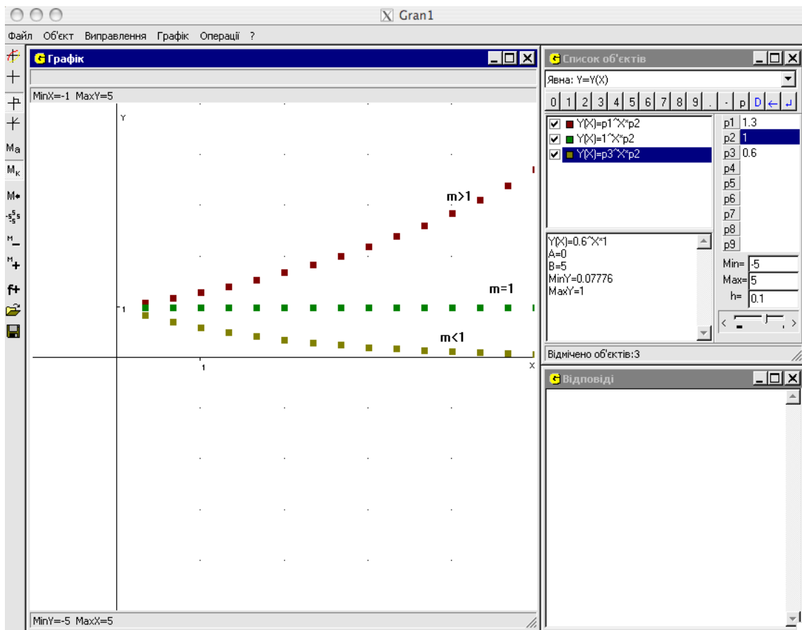
Рис.4.29. Види графіків для лінійної моделі.
