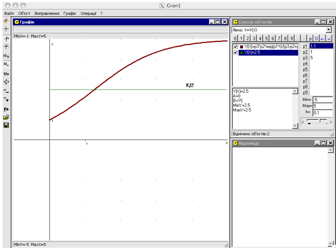
Рис. 4.38. Після інтенсивного зростання швидкість зростання чисельності популяції прямує до нуля.
