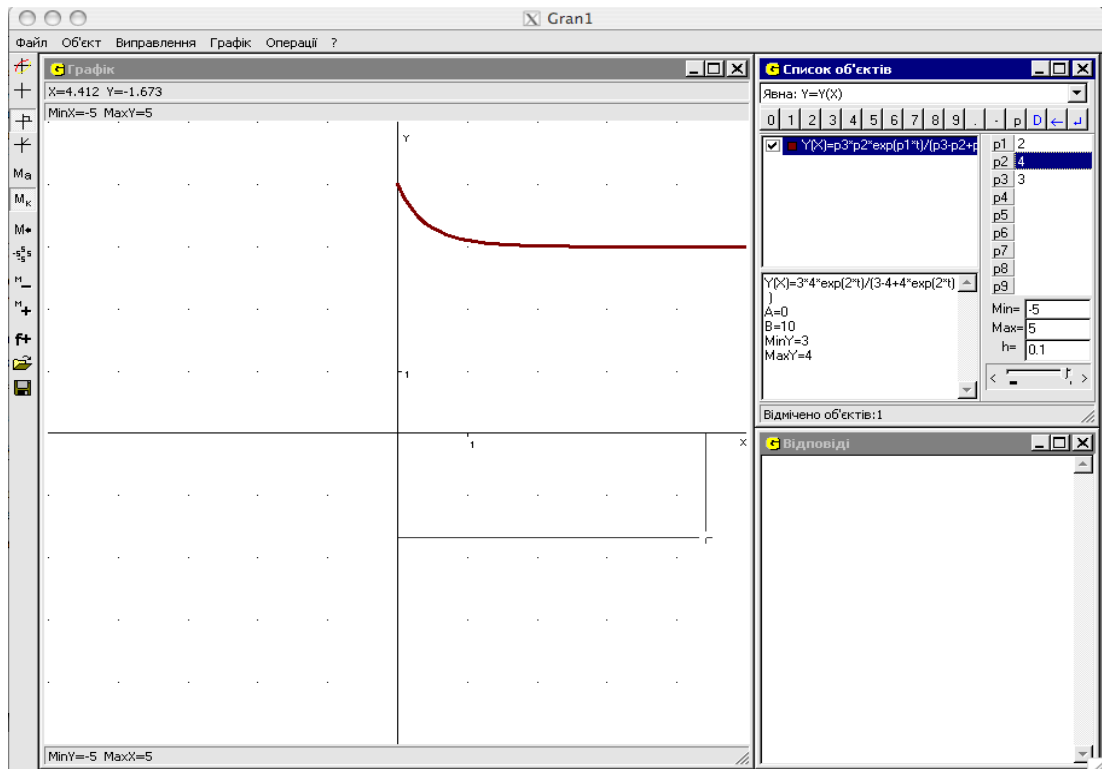
Рис. 4.36. Чисельність популяції зменшується до демографічної ніші.
