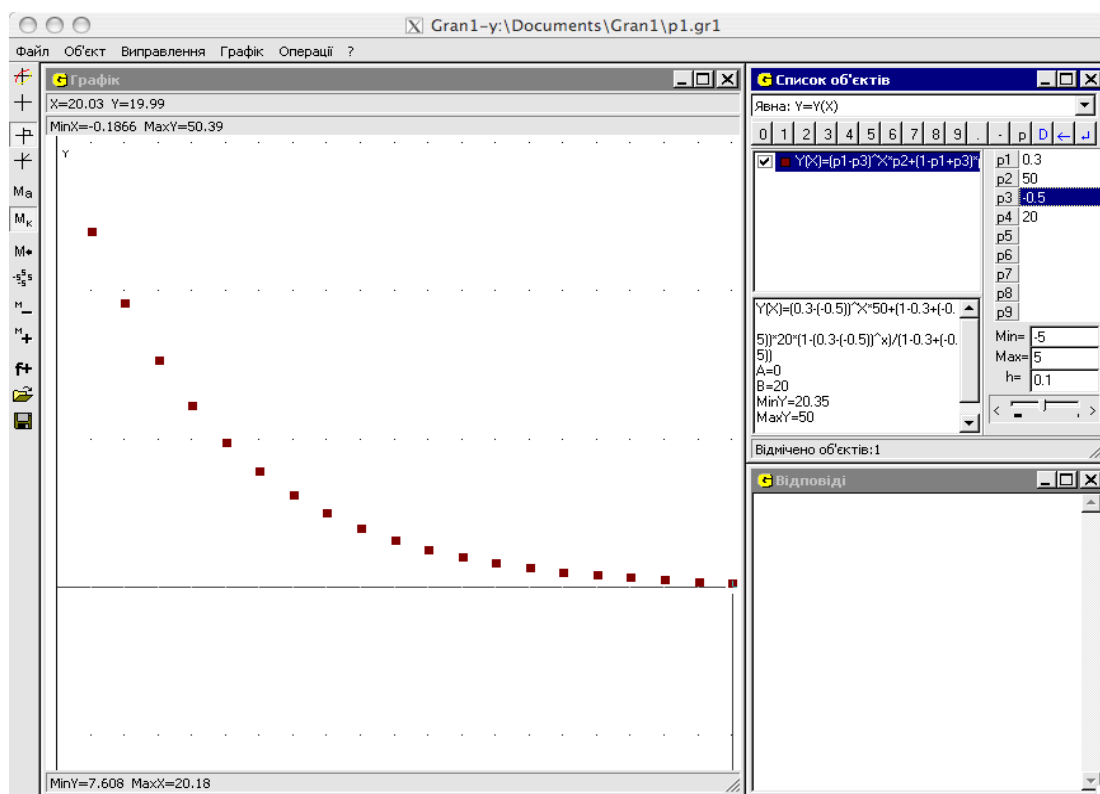
Рис. 4.31. Монотонне наближення чисельної популяції до значення рівноваги.
