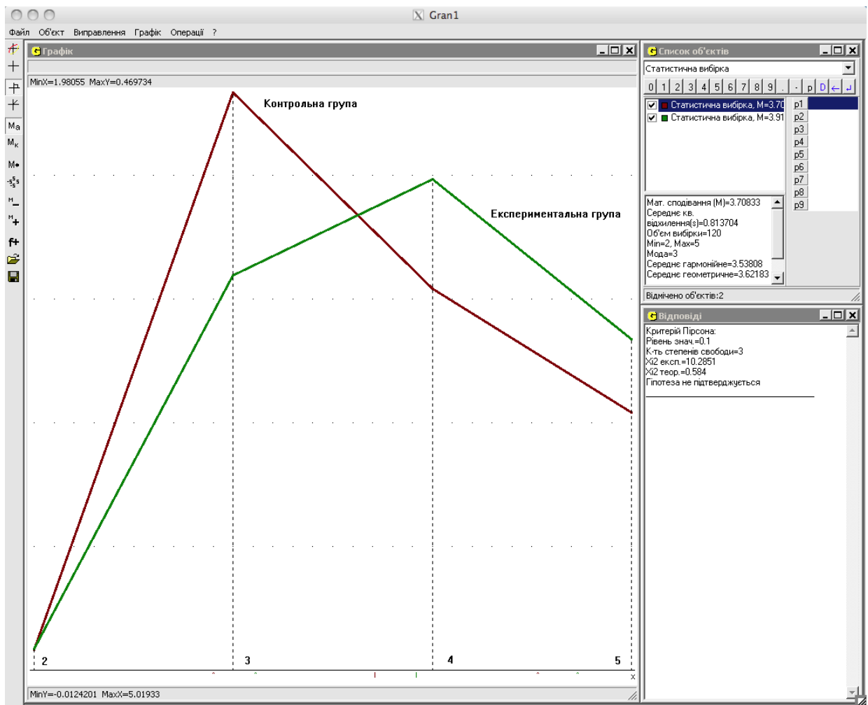
Рис. 4.39. Результати першої частини експерименту.
