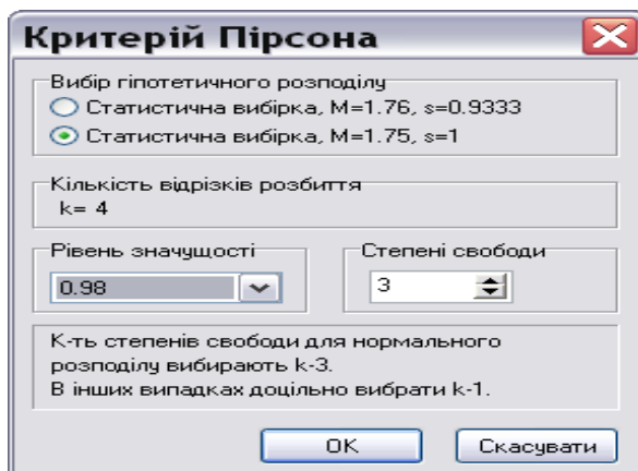
Рис. 4.17. Введення параметрів Критерію Пірсона.
