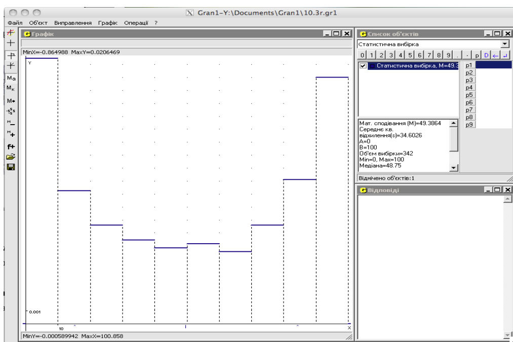
Рис. 4.14. Гістограма до Задачі 4.18.
