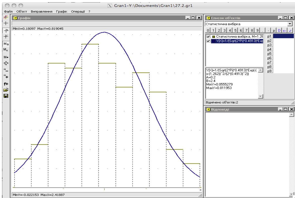
Рис. 4.16. Відповідь до Задачі 4.24.
