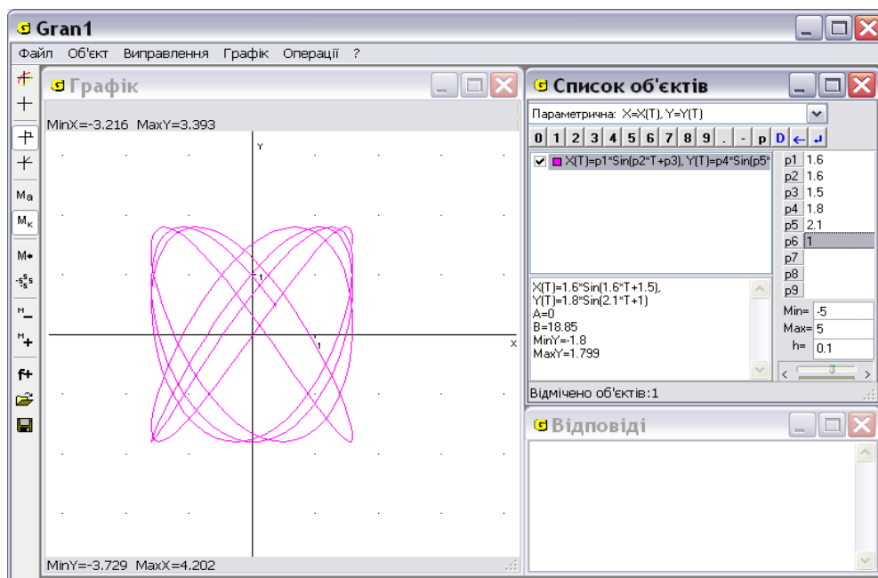
Рис. 2.23. Фігури Ліссажу.
