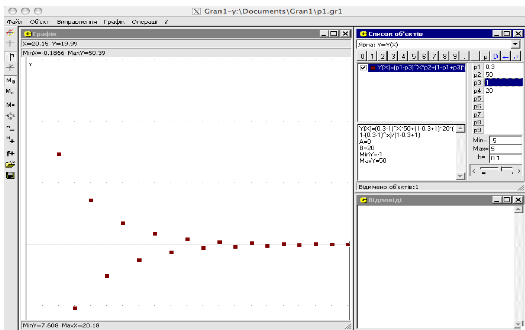
Рис. 4.32. Немонотонне наближення чисельної популяції до значення рівноваги.
