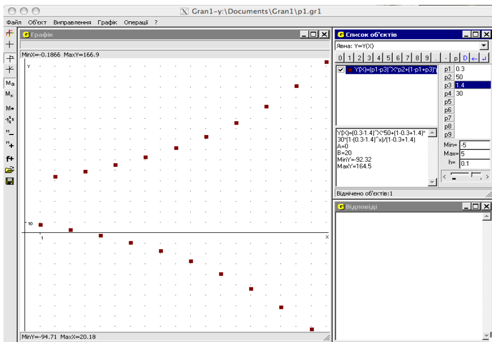
Рис. 4.34. Чисельність популяції по черзі то збільшується, то зменшується.
