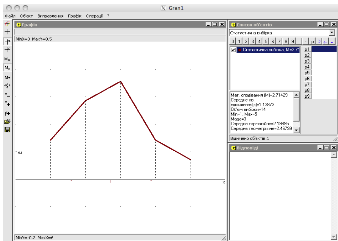
Рис.2.28. Полігон.
