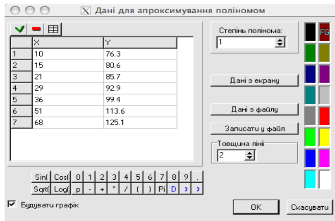
Рис. 4.22. Введення даних до Задачі 4.38.
