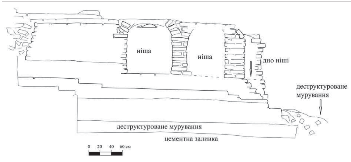
Лл. 11. Розріз В-В1 (через північно-східну стіну)
