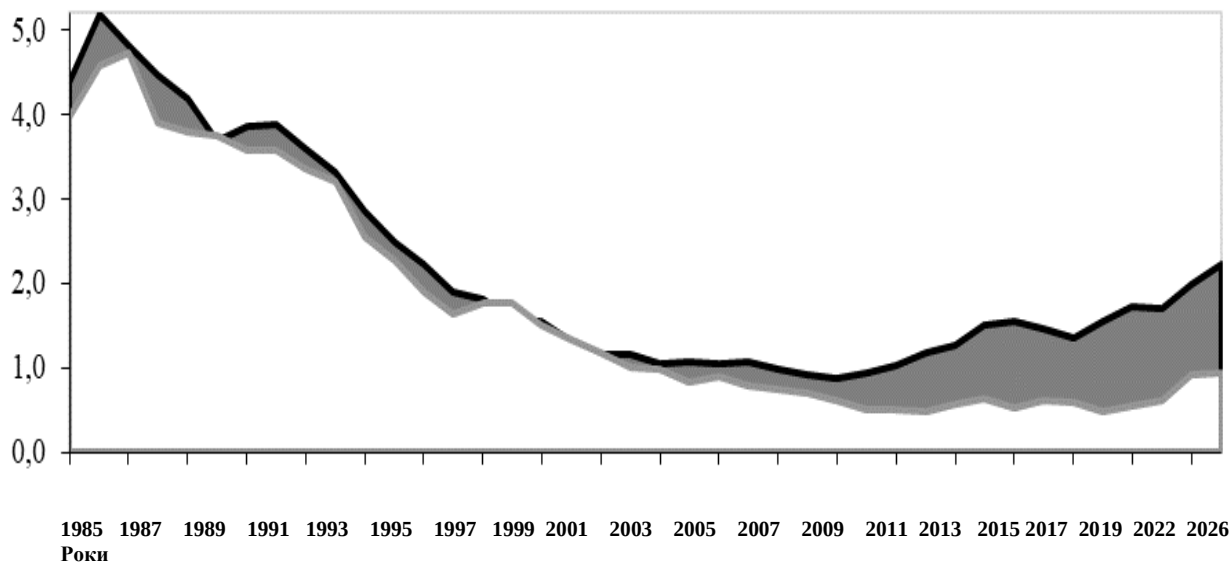
Рис. 32 Індеси радіального приросту сосни звичайної з використанням функції кубічного сплайна програмою ARSTAN – 20215 в лісорослинних умовах А 2-3 , В 2-3 Філії «Овруцьке спеціалізоване лісове господарство» ДП «Ліси України»
