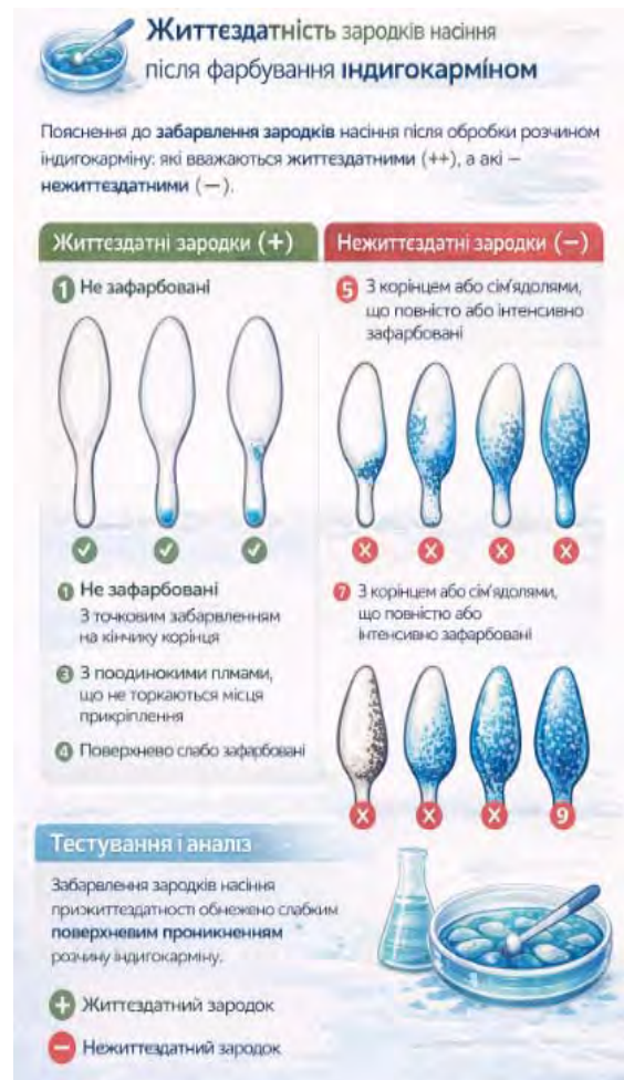
Рис. 6.1. Метод індигокарміну
