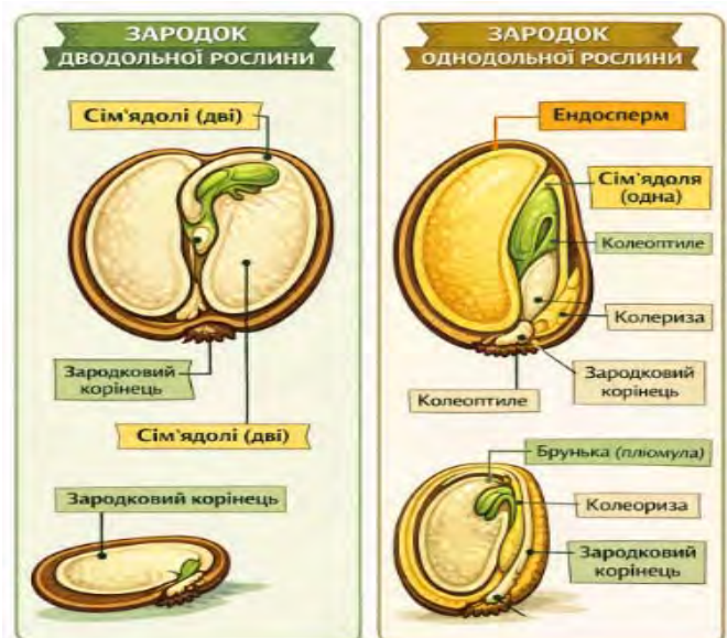
Рис. 1.24. Будова зародка
