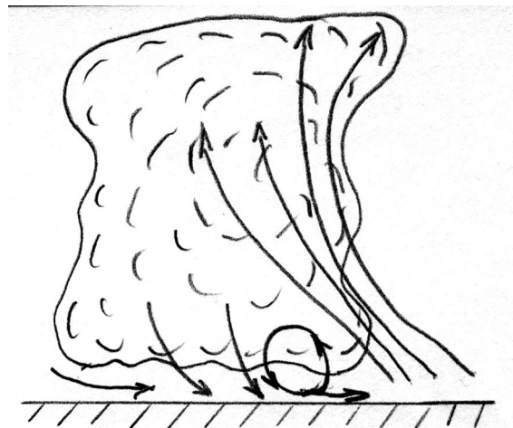
Мал. 6.37. Схема утворення шквалу.
