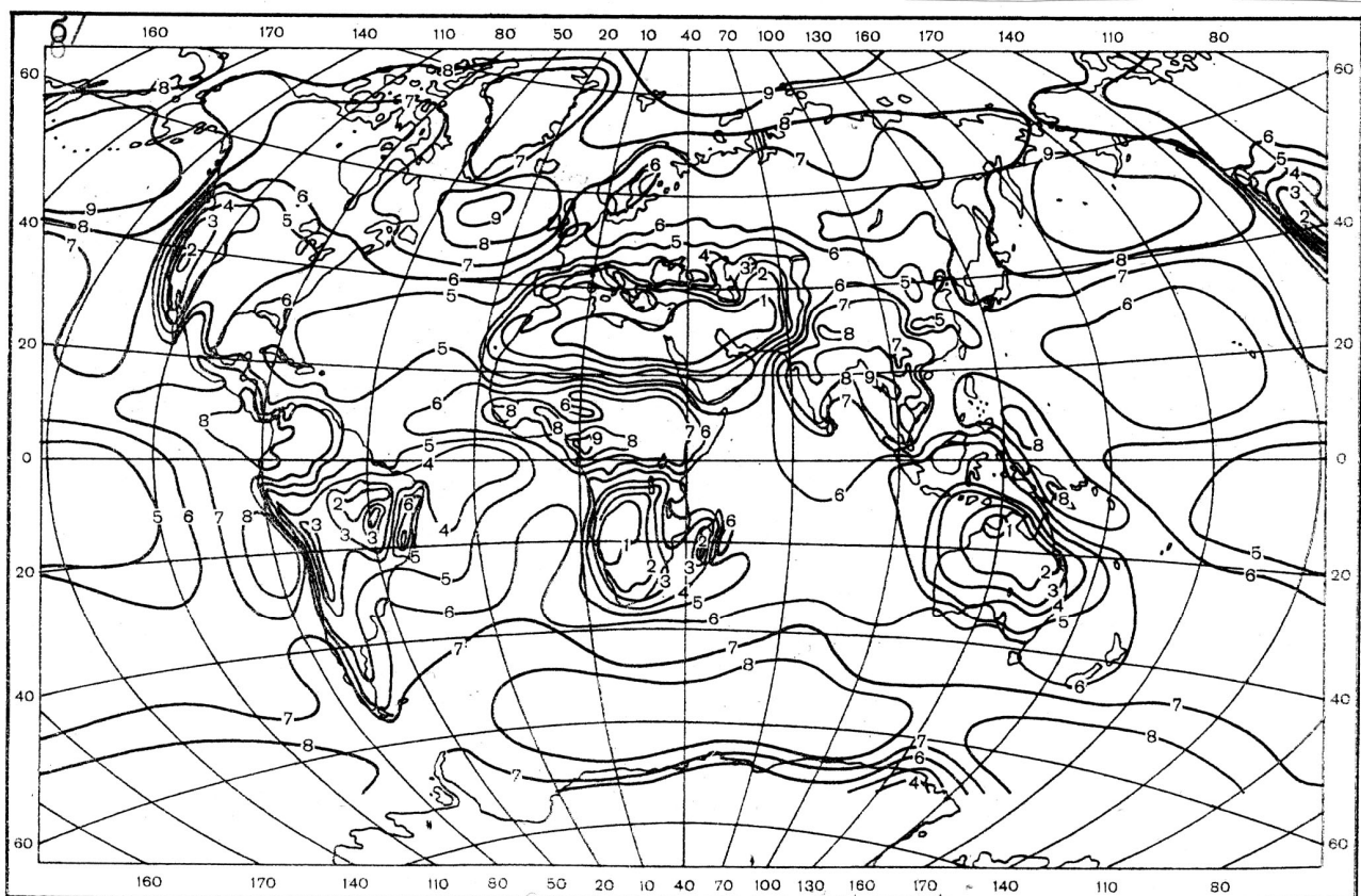
Мал. 5.7. Географічний розподіл середньої місячної хмарності (бали): а) – січень, б) – липень.
