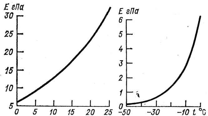
Мал. 5.1. Тиск насиченої водяної пари залежно від температури.
