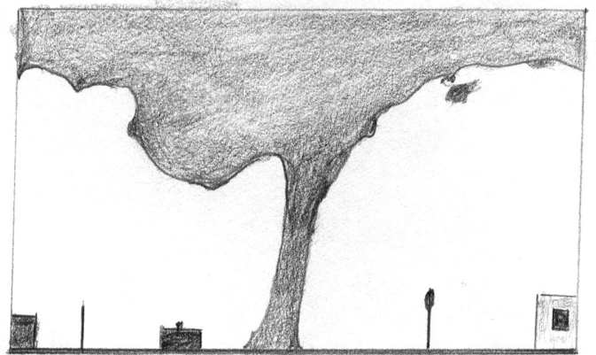
Мал. 6.38. Тромб, (торнадо)
