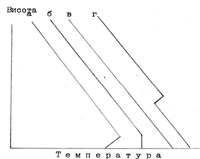
Мал. 4.9. Типи розподілу температури повітря з висотою (криві стратифікації): а – приземна інверсія, б – ізотермія, в – нормальний стан тропосфери, г – висотна інверсія.
