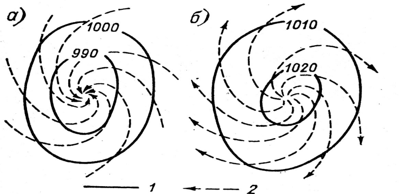
Мал. 6.18. Ізобари (1) та траєкторії перенесення повітря (2) в приземних шарах циклону (а) та антициклону (б).
