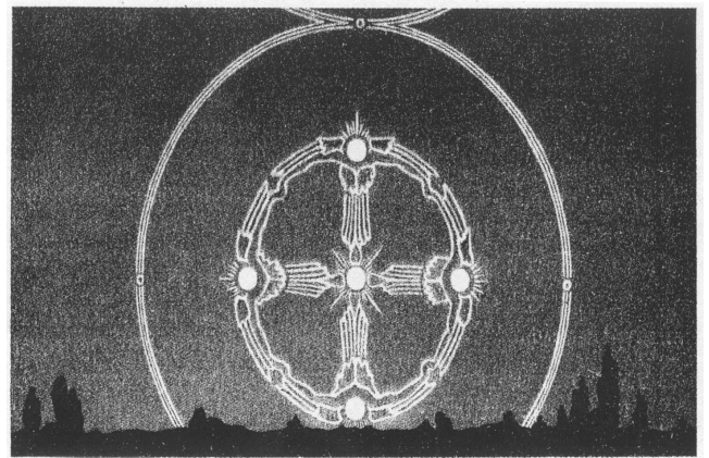
Мал. 5.6. Сонячний хрест у хмарах.
