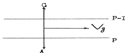
Мал. 6.12. Геострофічний вітер
