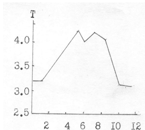
Мал. 3.4. Річний хід чинника мутності атмосфери.
