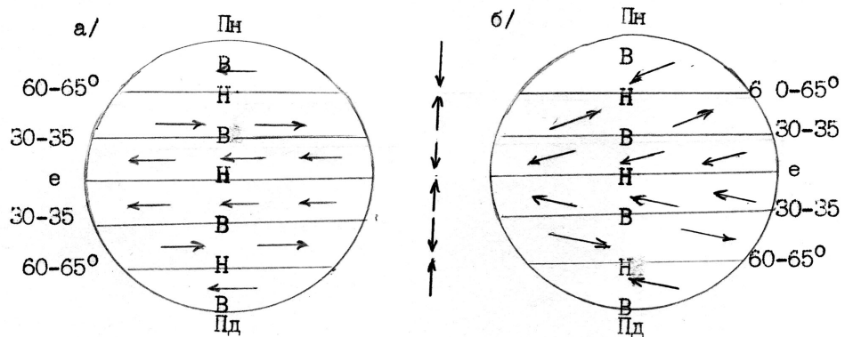
Мал. 6.26. Схема зонального розподілу атмосферного тиску та повітряних течій у нижній тропосфері вище шару тертя (а) та в шарі тертя (б)
