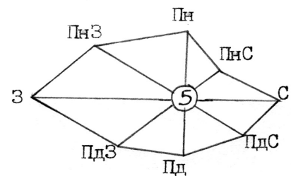
Мал. 6.10. Напрямок вітру в румбах та градусах.
