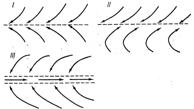
Мал.6.30. Основні типи течій повітря в зоні конвергенції в середині тропічних широт I – сходження течій на тропічному фронті поблизу екватора, II - сходження течій на значній відстані від екватора (літній екваторіальний мусон), III – екваторіальна зона західних вітрів.
