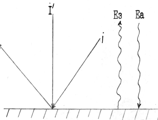
Мал. 3.6. Складові частини радіаційного балансу.
