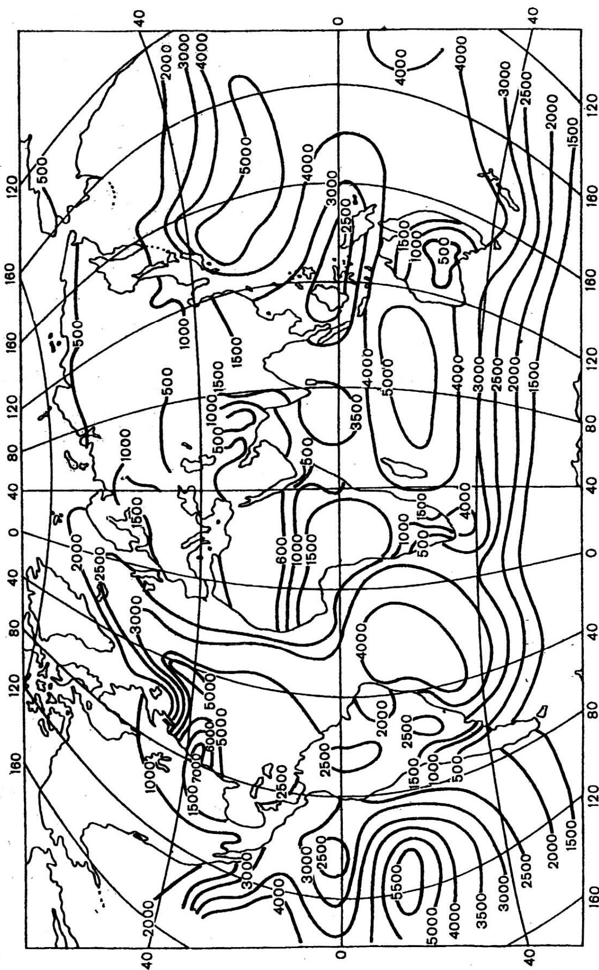
Мал. 4.2. Річні витрати тепла на випаровування вологи ( \text{МДж/м}^2 )
