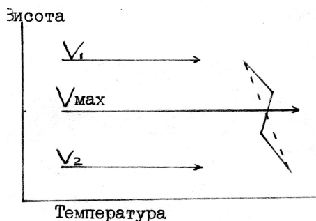
Мал. 4.10. Формування динамічної інверсії.
