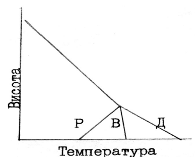
Мал. 4.12. Добовий хід стратифікації атмосфери над суходолом: Р – ранок, В – вечір, Д – день.
