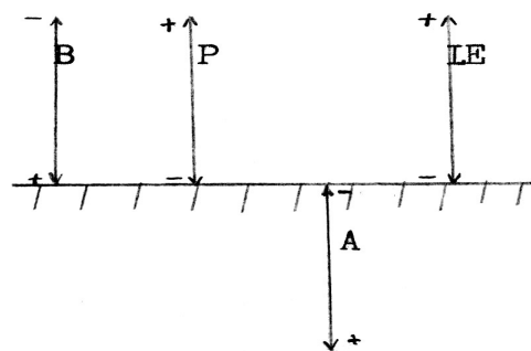
Мал. 4.1. Складові теплового балансу земної поверхні.
