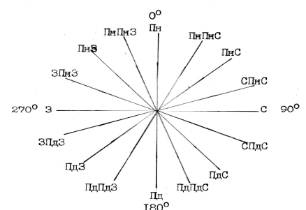
Мал. 6.11. Роза вітрів.
