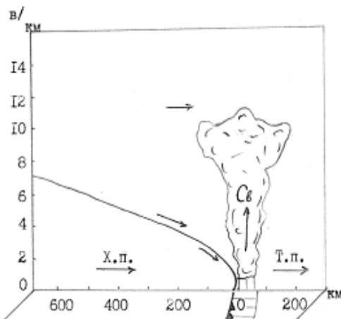
Мал. 6.20. Вертикальний розріз теплового (а) та холодного (б, в) фронтів з системами хмар та опадів.
