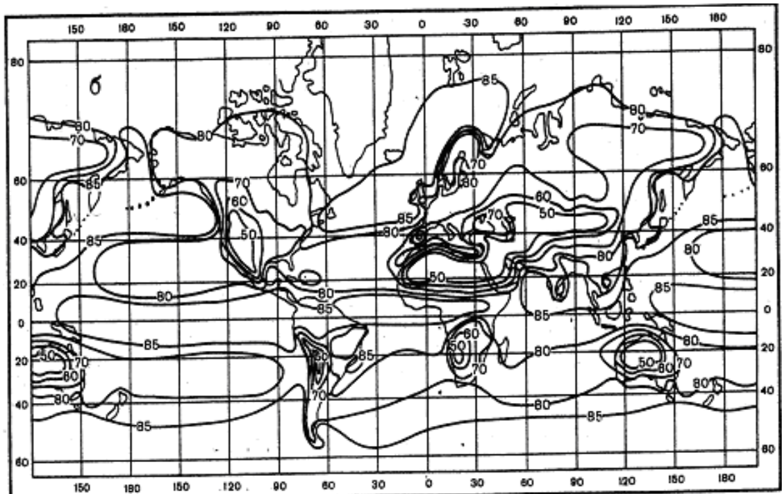
Мал. 5.5. Середній багаторічний розподіл відносної вологості повітря (%): а) – січень, б) – липень.
