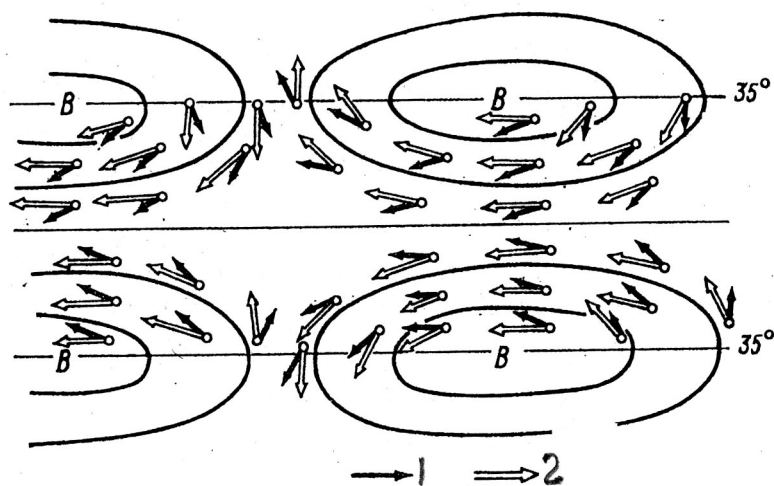
Мал. 6.29. Схема течій повітря в зоні пасатів 1 – вітри біля земної поверхні, 2 – над шаром тертя.
