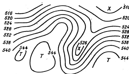
Мал. 6.6. Области тепла (Т) та холоду (Х) на карті відносної баричної топографії ізобаричної поверхні 500 гПа над поверхнею 1000 гПа
