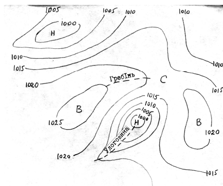
Мал. 6.2. Баричні системи на синоптичній карті: H - циклон, B - антициклон, C - сідловина.
