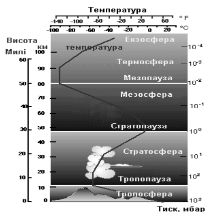
Мал. 2.1. Вертикальний розріз атмосфери. Ламана крива – особливості зміни температури в різних шарах атмосфери.
