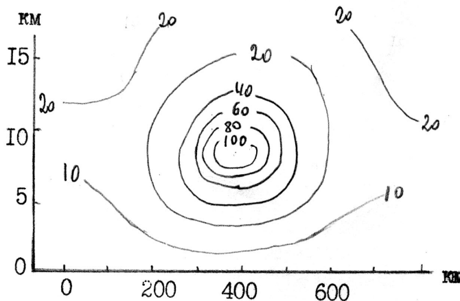
Мал. 6.22. Поперечний перетин струминної течії, м/с
