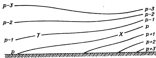
Мал. 6.5. Вертикальний розріз ізобаричних поверхонь в районах тепла (Т) та холоду (Х)
