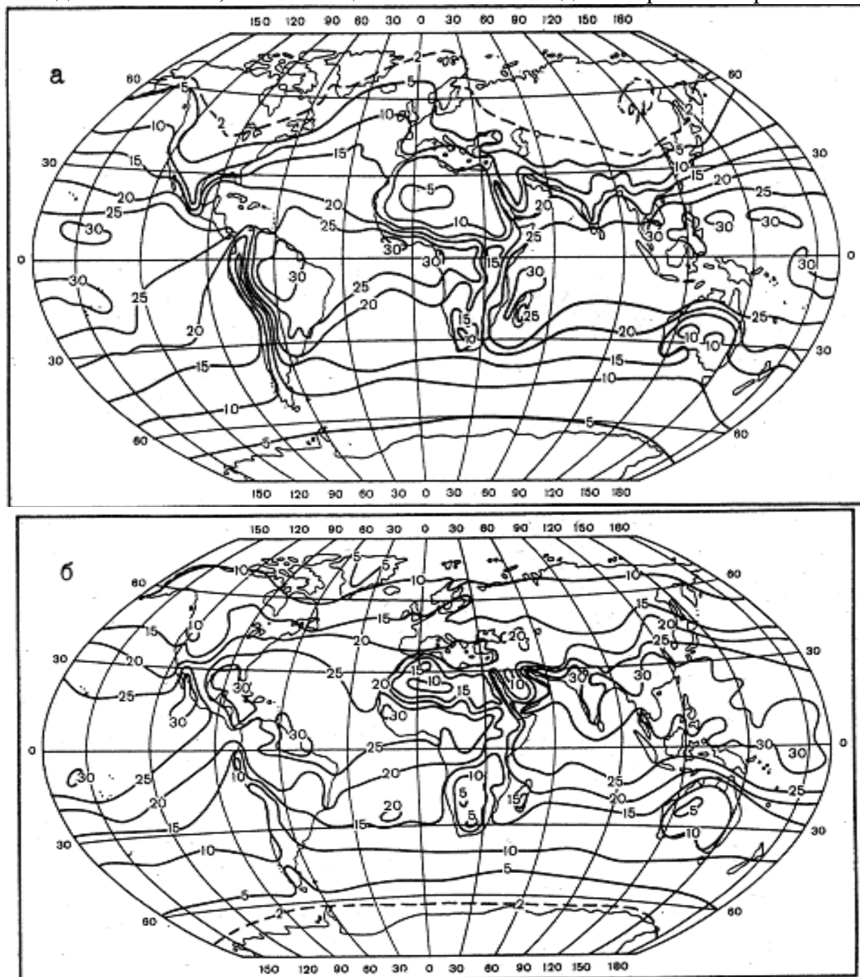
Мал. 5.4. Середній багаторічний розподіл парціального тиску водяної пари (гПа): а) – січень, б) – липень.
