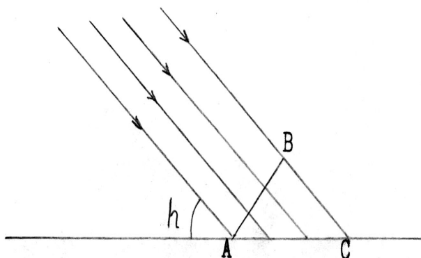
Мал. 3.2. Надходження прямої сонячної радіації на перпендикулярну до променів поверхню (AB) та на горизонтальну поверхню (AC).
