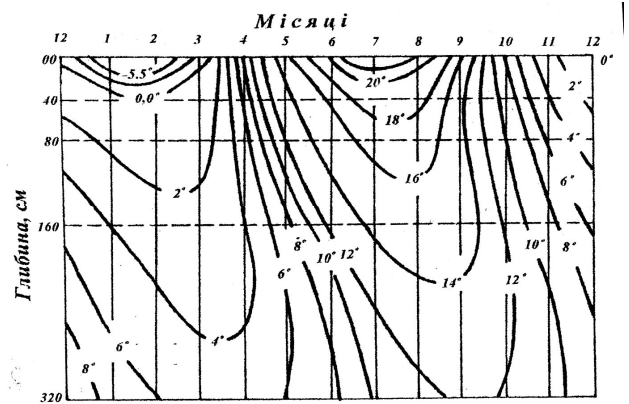
Мал. 4.4. Термоізоплети річного ходу температури ґрунту в Житомирі.
