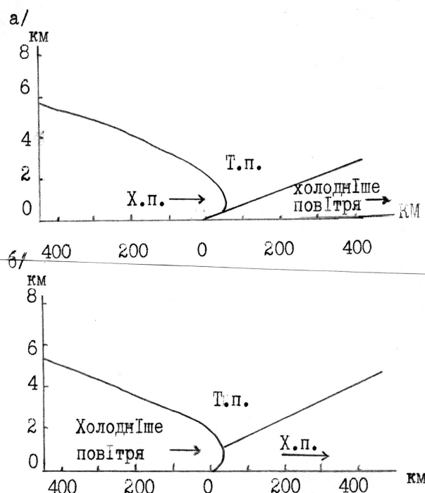
Мал. 6.21. Фронти оклюзії: за типом теплового фронту (а) та за типом холодного фронту (б)
