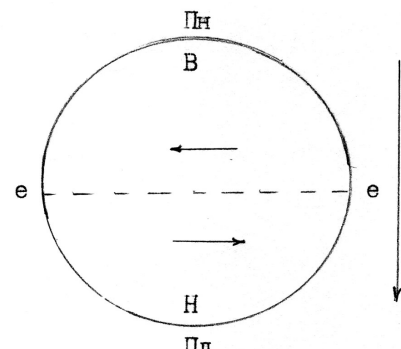
Мал. 6.28. Схема зонального розподілу тиску та течій повітря вище 20 – 25 км, коли у північній півкулі літо.
