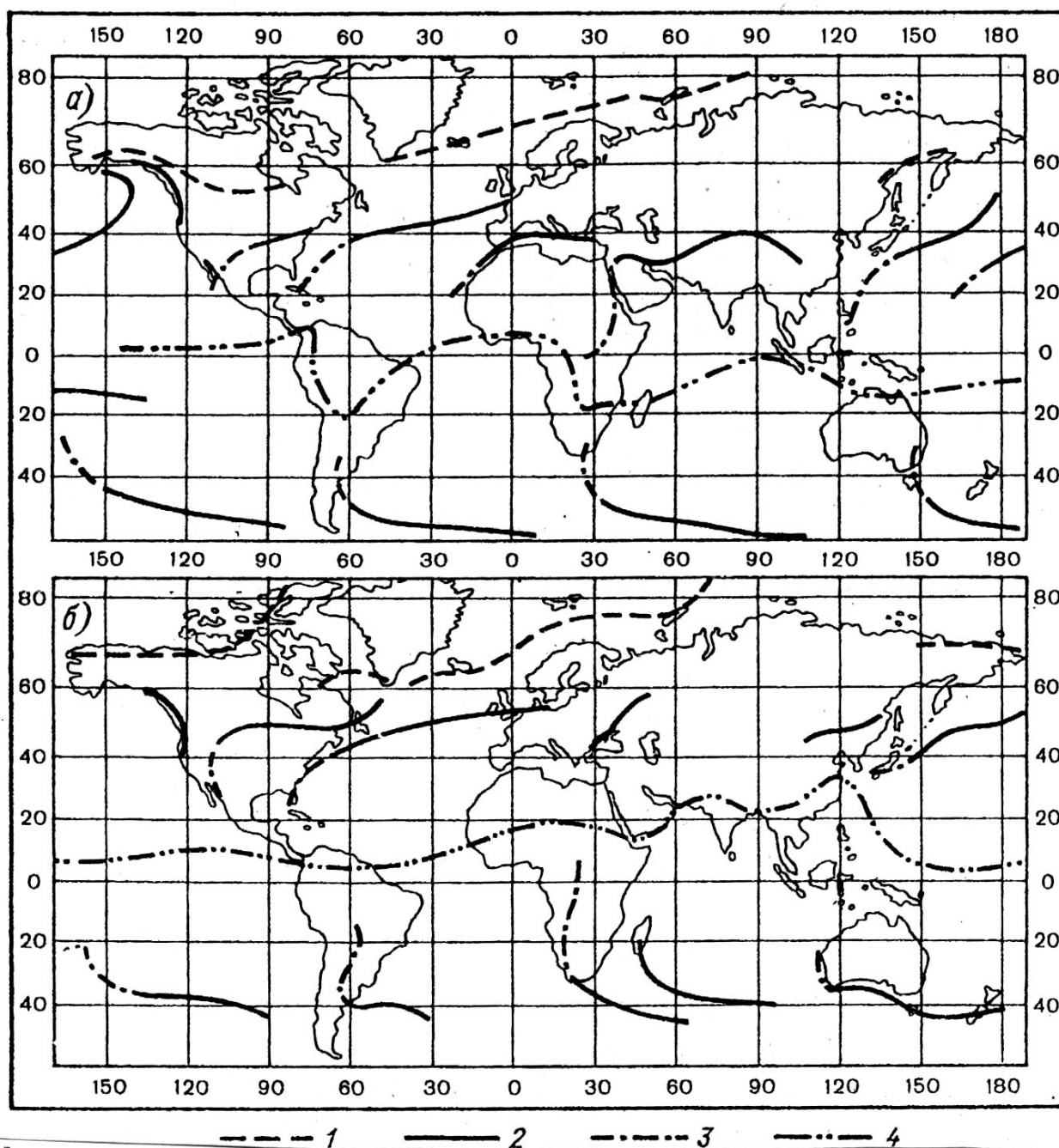
Мал. 6.25. Кліматологічні fronti: а) – січень, б) – липень. 1 – арктичний, 2 – полярний, 3 – пасатний (продовження полярного фронту в зону тропіків), 4 – тропічний.
