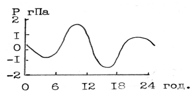
Мал. 6.9. Середній добовий хід атмосферного тиску в тропічних широтах Індійського океану
