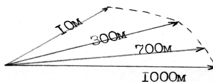
Мал. 6.16. Вітер у шарі тертя.
