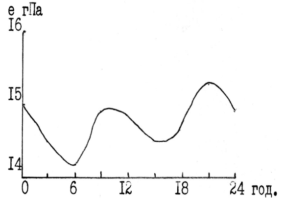
Мал. 5.3. Добовий хід тиску водяної пари у Житомирі в липні.
