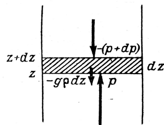
Мал. 6.1. Сили, що діють на елементарний об'єм повітря
