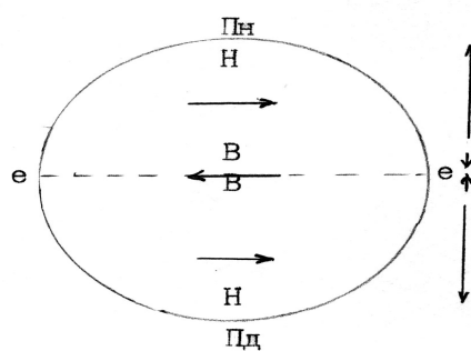
Мал. 6.27. Схема зонального розподілу тиску і течій повітря у верхній тропосфері і нижній стратосфері.
