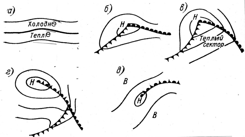
Мал. 6.33. Схема розвитку фронтальних циклонів а, б) – стадії хвилі, в) – молодий циклон, г, д) – стадії оклюзії.
