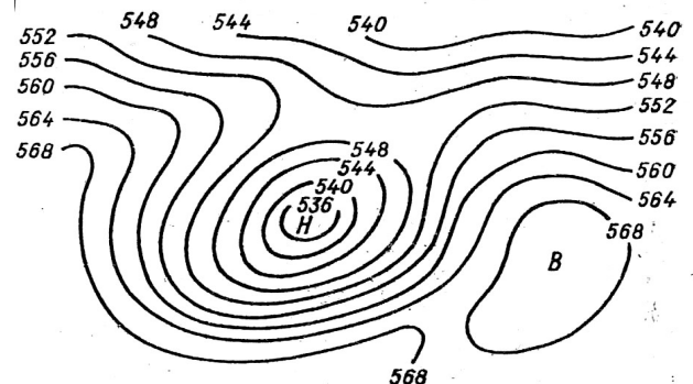
Мал. 6.4. Циклон (Н) та антициклон (В) на карті абсолютної топографії ізобаричної поверхні 500 гПа
