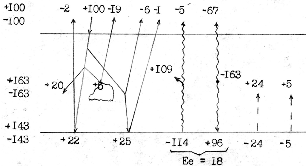
Мал. 4.13. Тепловий баланс Землі, земної поверхні та атмосфери
