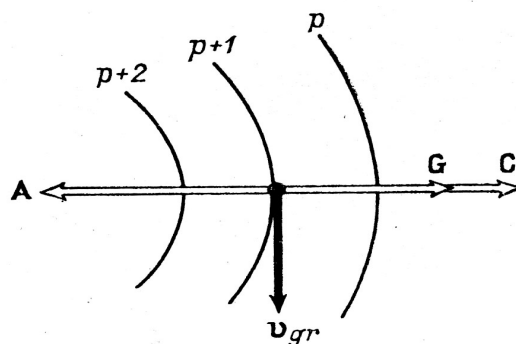
Мал. 6.14. Градієнтний вітер в антициклоні: G – сила баричного градієнта, A – відхиляюча сила обертання Землі, C – відцентрова сила, V_{gr} – градієнтний вітер.
