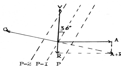
Мал. 6.17. Графік зміни напрямку та швидкості вітру в шарі тертя (спіраль Екмана).
