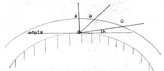
Мал. 3.3. Шлях сонячного променя в атмосфері за різної висоти Сонця над обрієм
