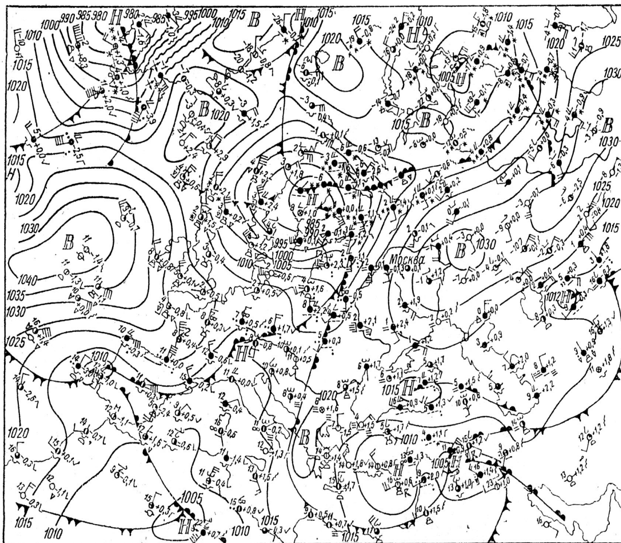
Мал. 6.39. Синоптична карта.
