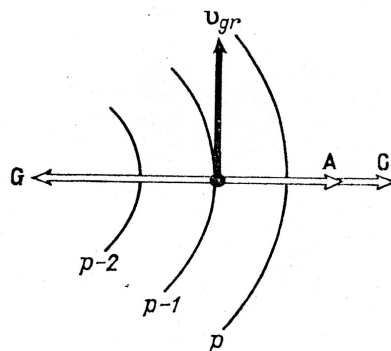
Мал. 6.13. Градієнтний вітер в циклоні: G – сила баричного градієнта, A – відхиляюча сила обертання Землі, C – відцентрова сила, V_{gr} –
