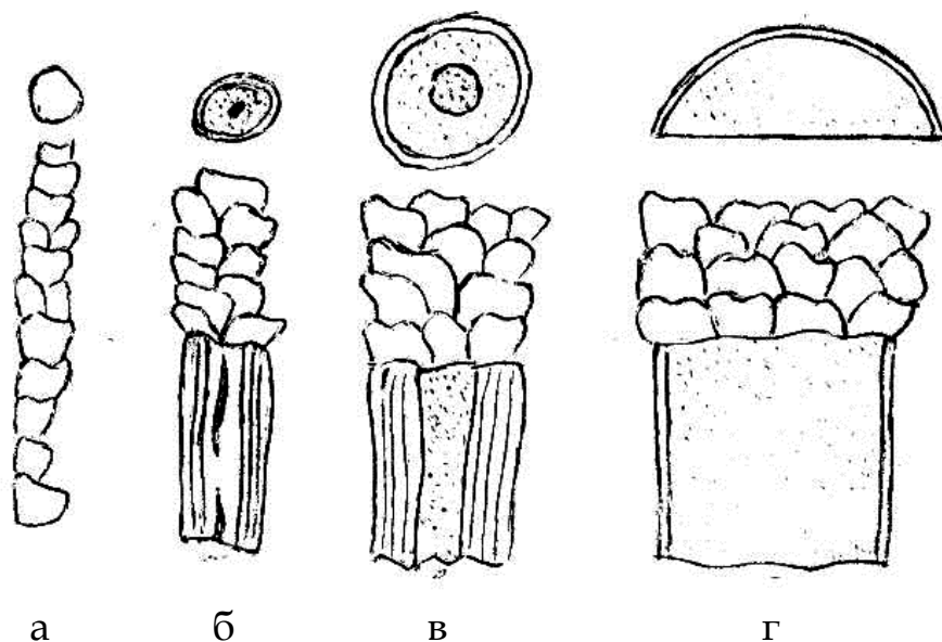
Рис. 3.6. Поздовжній вигляд та поперечний переріз волокон вовни:
