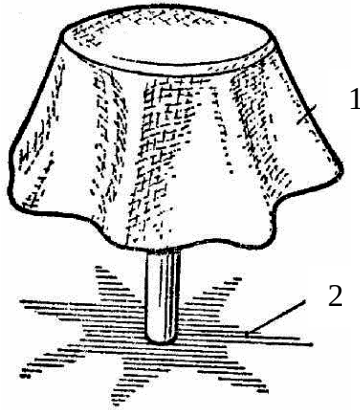
Рис. 14.1. Визначення драпірувальності тканини дисковим методом:
