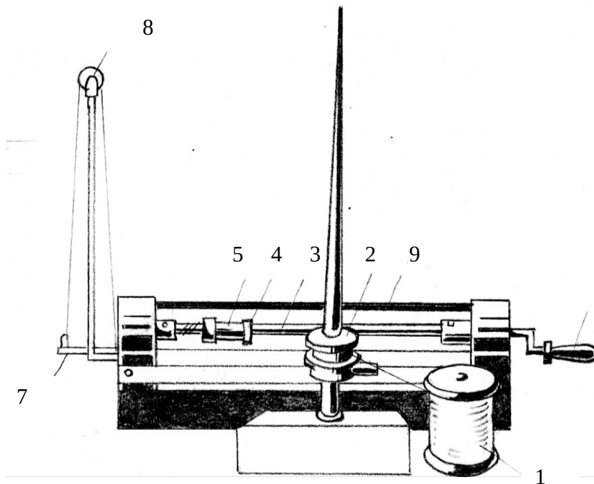
Рис. 4.2. Прилад ЦНІХБІ
