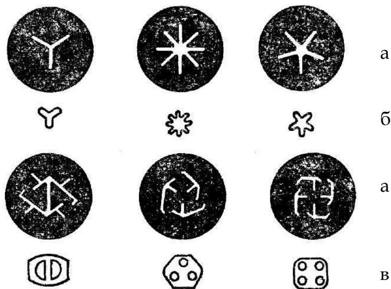
Рис. 7.1. Форми поперечного перерізу: а – профільованих отворів фільер; б – профільованих волокон; в – порожнистих волокон
