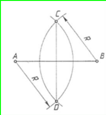
Рис. 13.1 Поділ відрізка на дві рівні частини Рис. 13.2 Поділ відрізка на довільне число рівних частин
