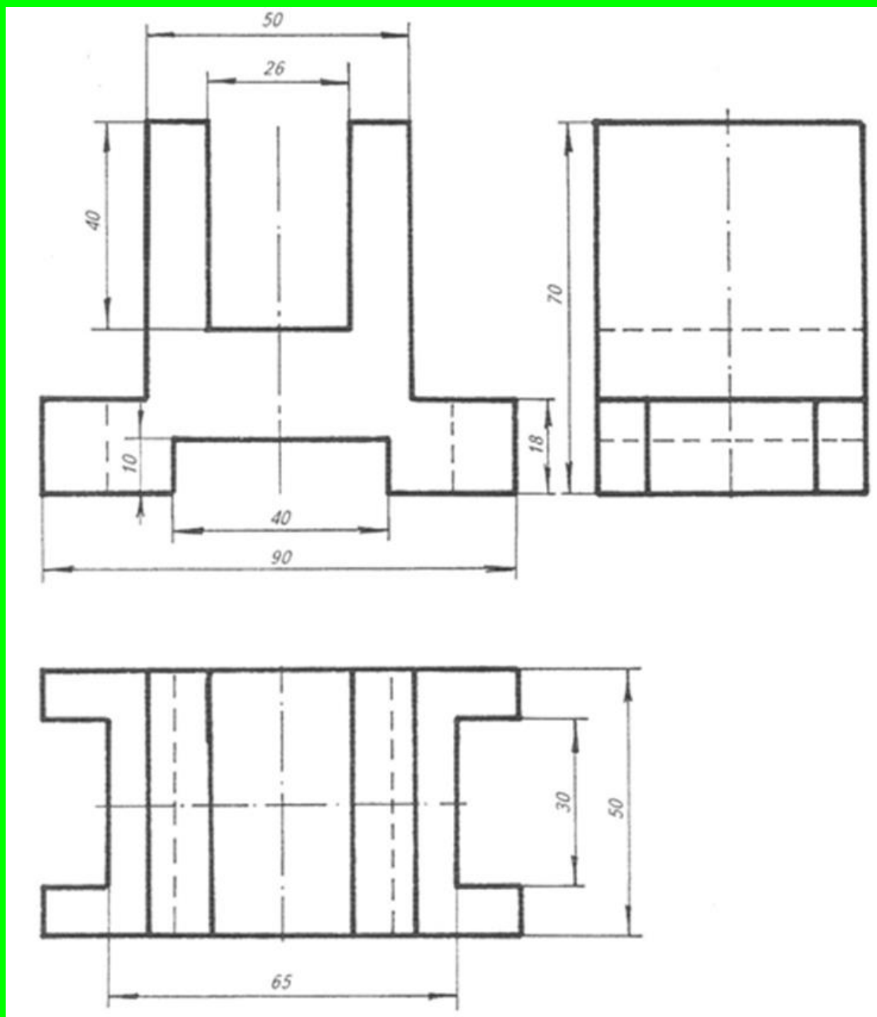
Рис.14.4 Зразок виконання графічних робіт № 14.1-14.2
