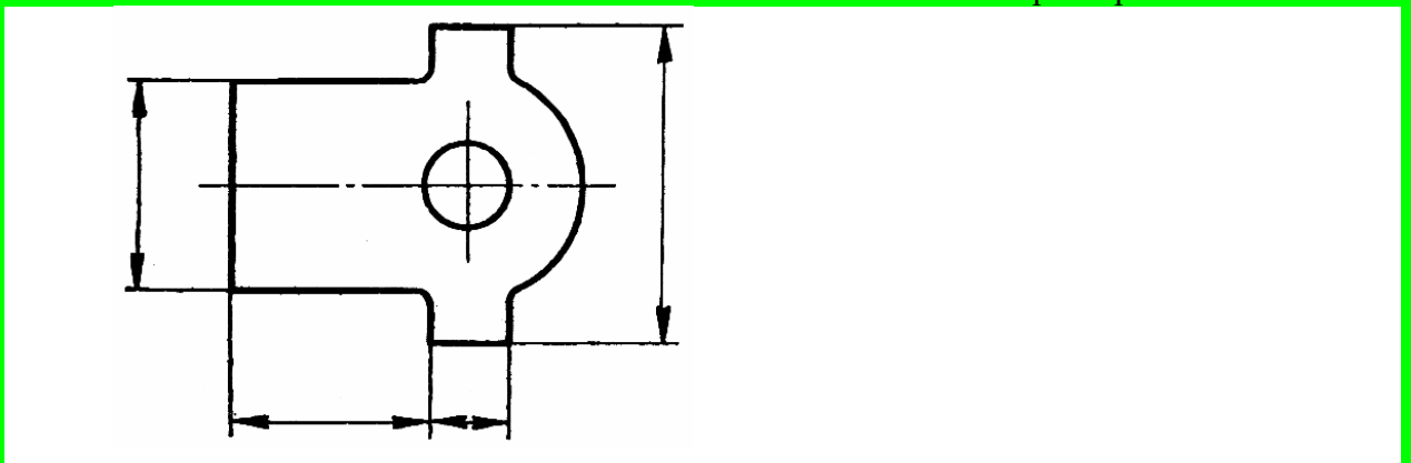
Рис.12.4 Відстань між розмірною лінією і контуром
