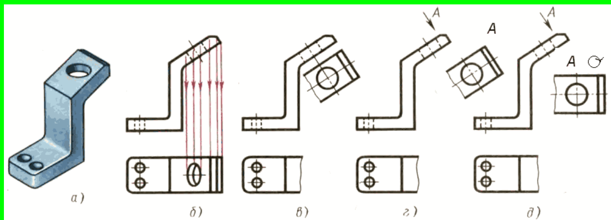
Рис. 14.3 Додаткові вигляди
