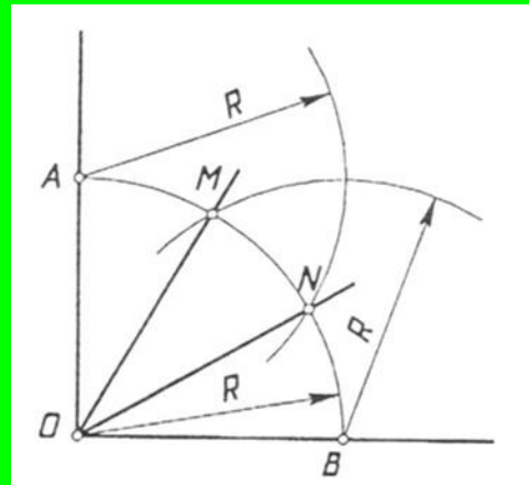
Рисунок 13.4 Поділ прямого кута на три рівні частини
