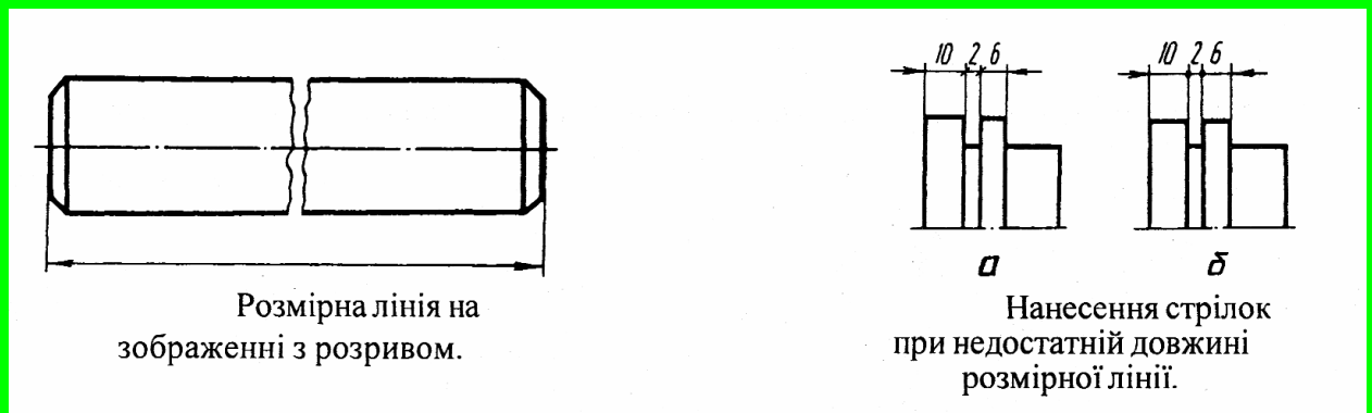
Рис. 12.8 Різні способи нанесення стрілок
