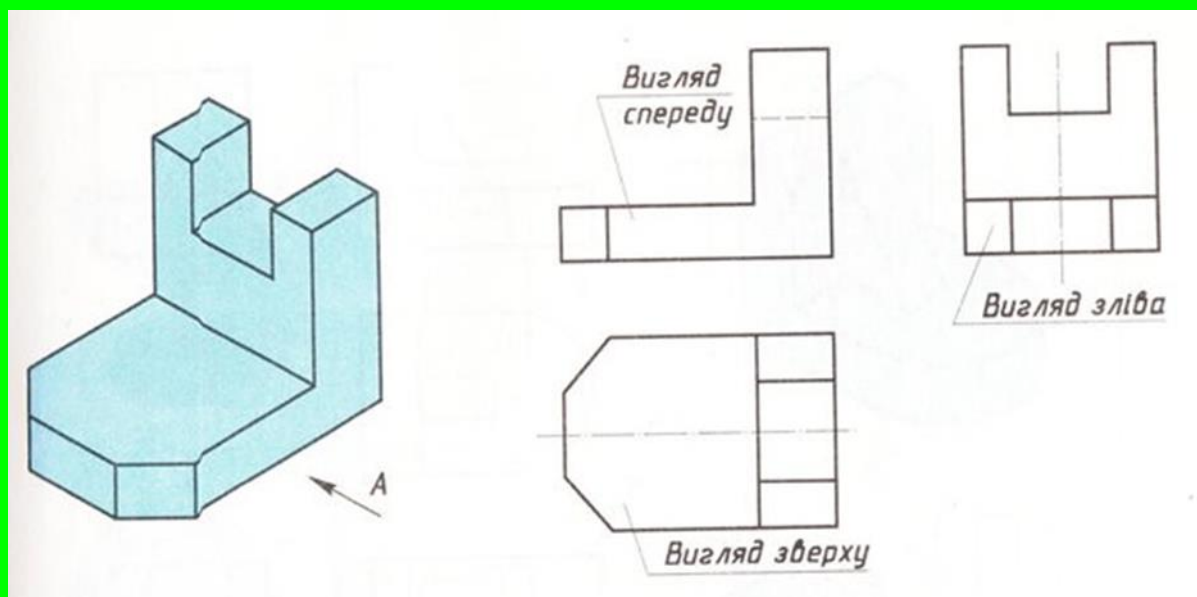
Рис.14.2 Побудова трьох основних виглядів деталі.
