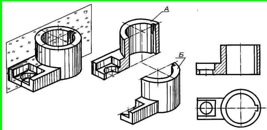
Рис. 15.4 Фронтальний розріз
