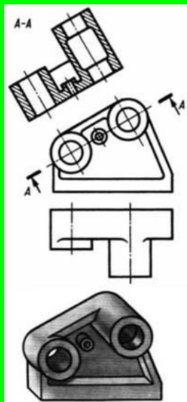
Рис. 15.5 Похилий розріз
