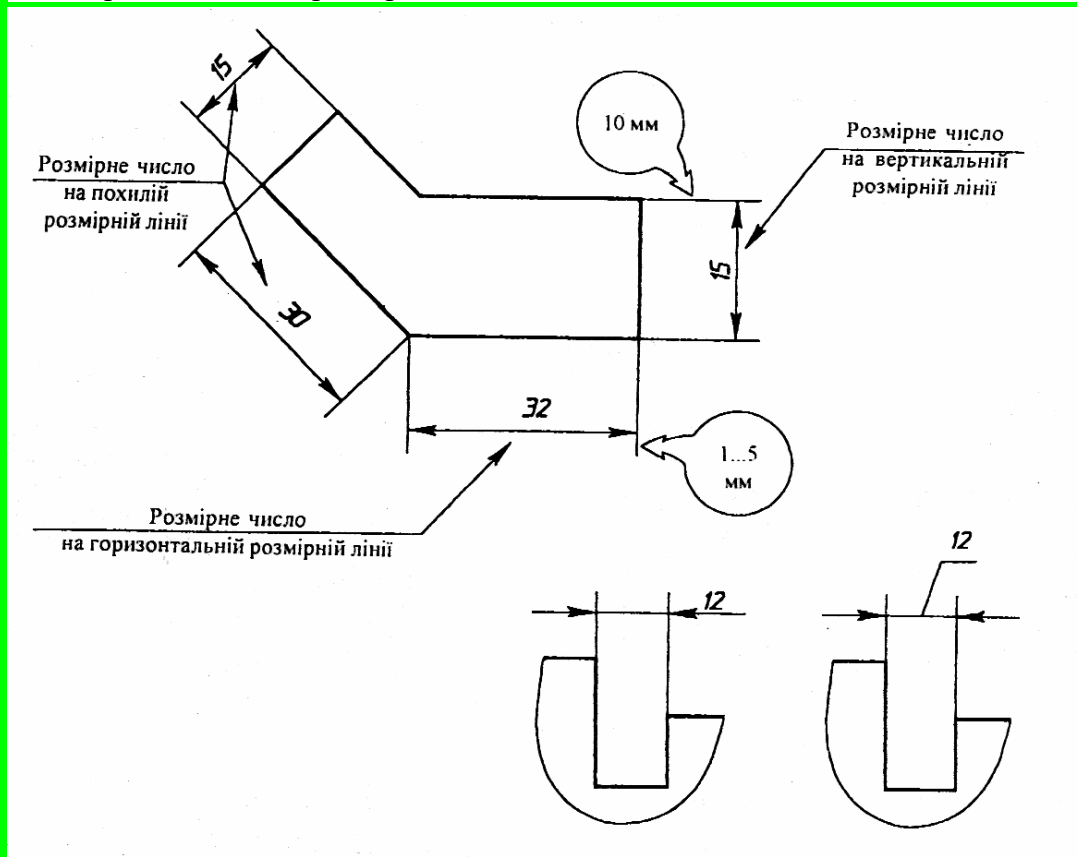
Рис12.6 Розмірні числа
