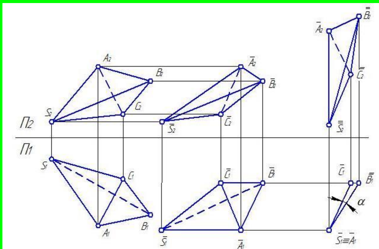
Рис. 6.1 Визначення розміру двогранного кута при ребрі AS .
