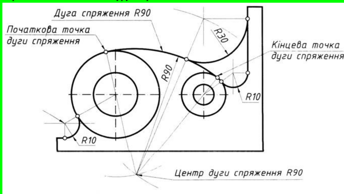
Рисунок 13.6 Кресленик деталі з елементами спряжень
