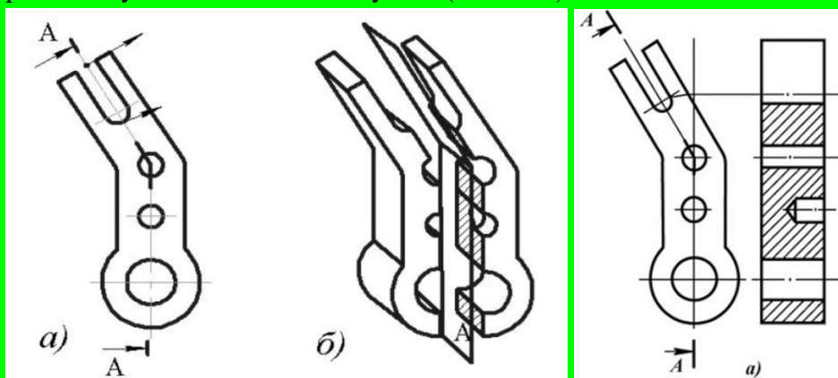
Рис. 7.12 Ламаний розріз
