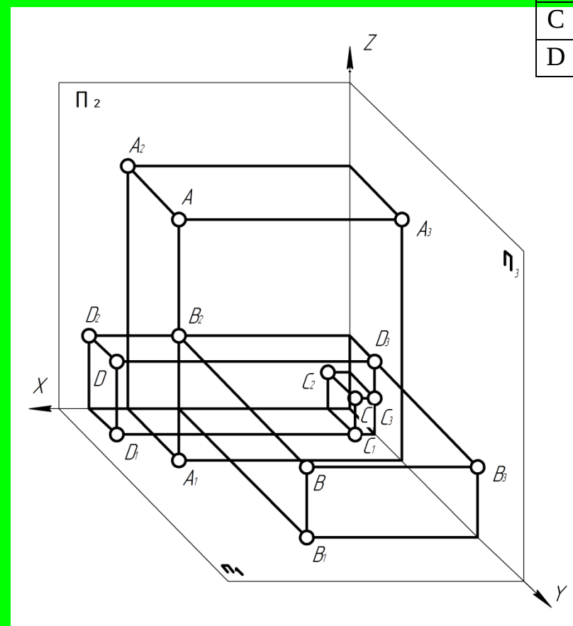
Рис.1.1 Просторове і комплексне зображення точки.
