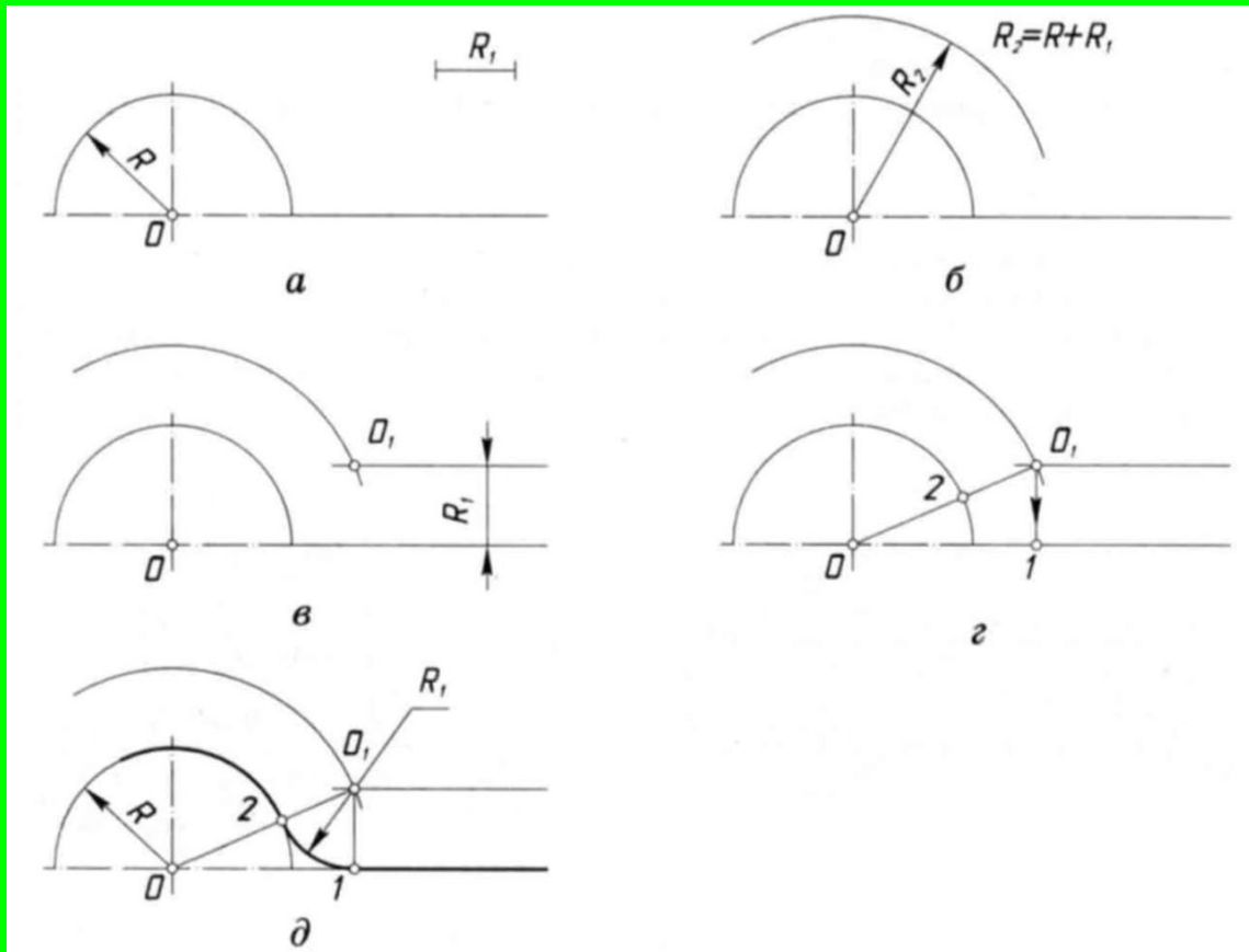
Рис. 13.11 Послідовність побудови спряження прямої і кола
