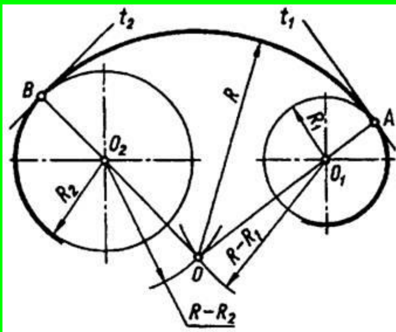
Рис. 13.13 Внутрішнє спряження
