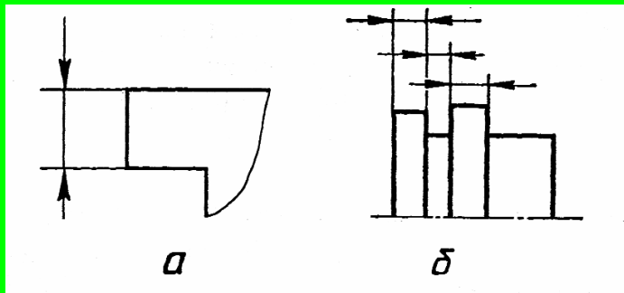
Рис.12.5 Розміщення стрілок зовні виносних ліній: а - для одного розміру; б – для декількох розмірів.
