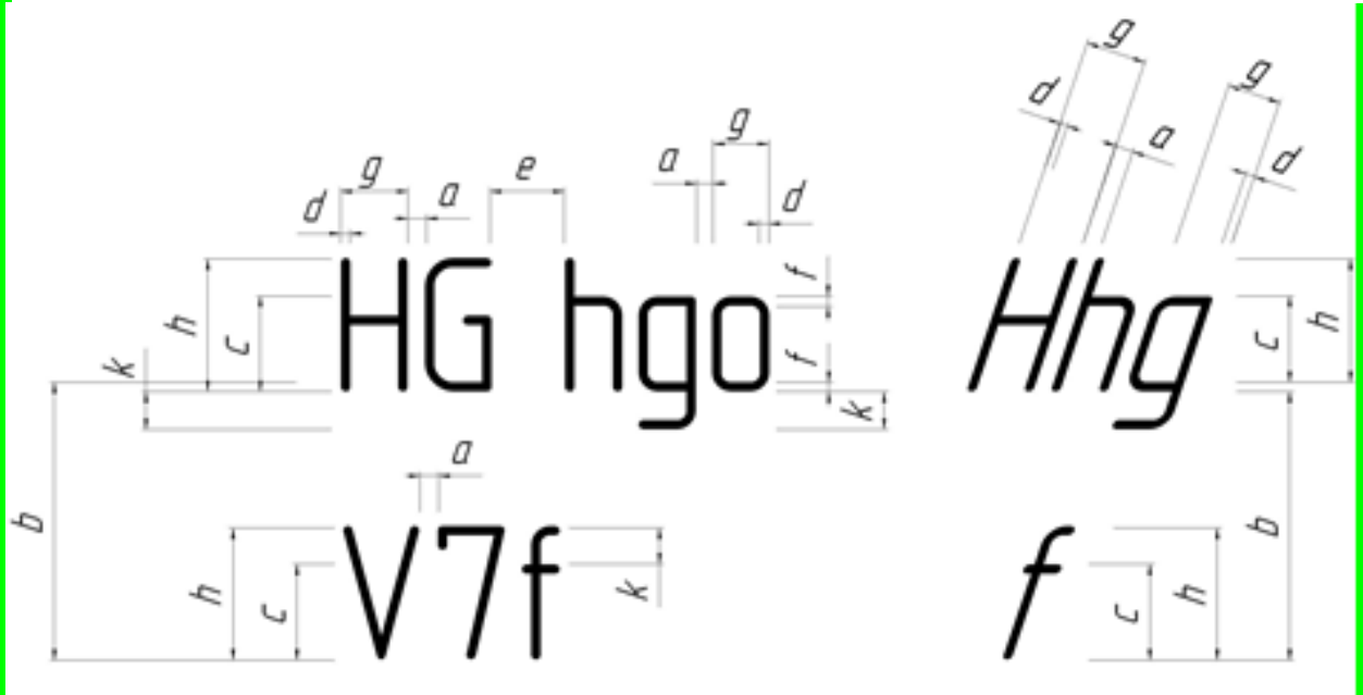
Рис. 11.1 Параметри креслярського шрифту
