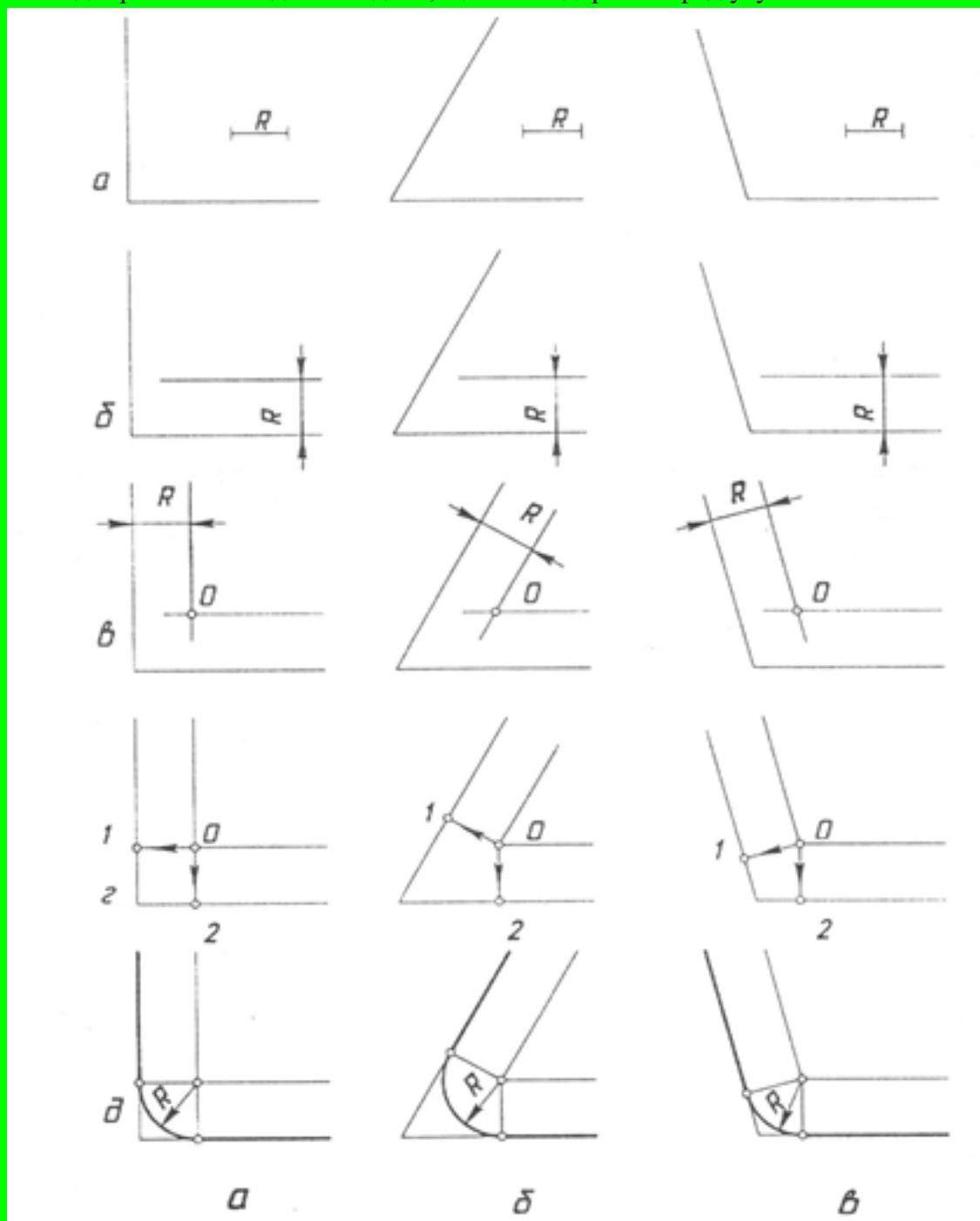
Рис.13.8 Послідовність виконання спряження двох прямих
