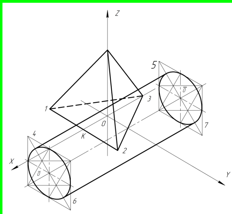
Рис. 3.6 Приклад побудови кола у прямокутній ізометричній проєкції
