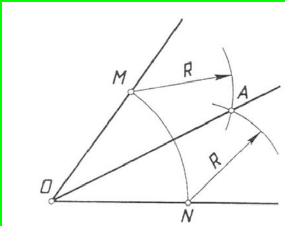
Рисунок 13.3 Поділ кута на дві рівні частини
