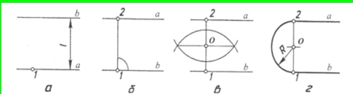
Рис. 13.9 Спряження паралельних прямих
