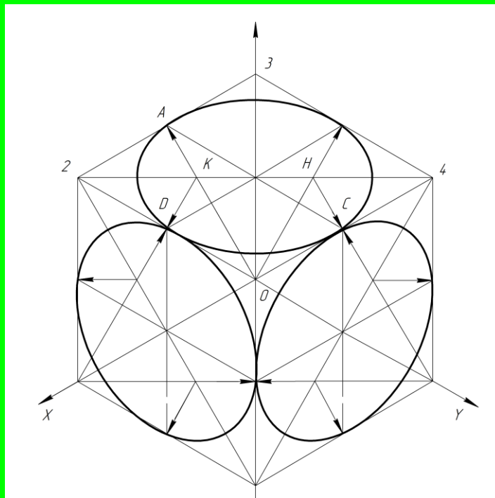
Рис. 3.6 Приклад побудови кола у прямокутній ізометричній проєкції
