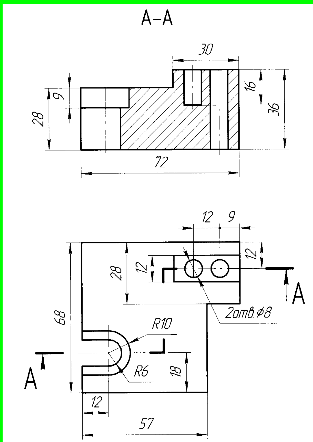
Рис.15.16 Приклад виконання графічної роботи №15.2
