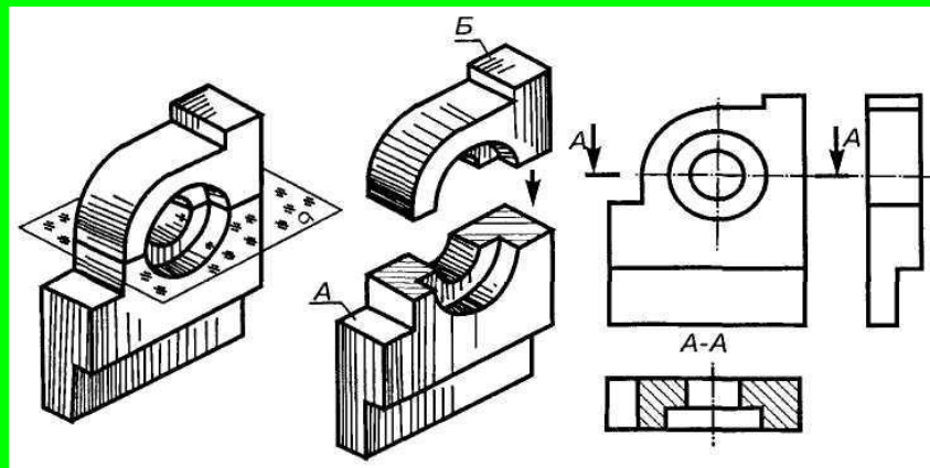
Рис. 15.3 Горизонтальний розріз
