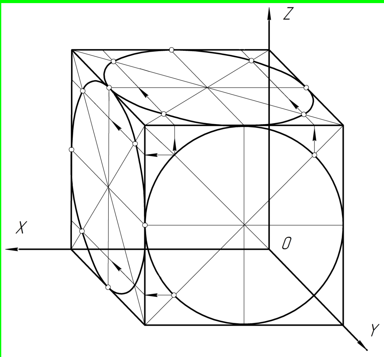
Рис. 3.5 Приклад побудови кола у фронтальній косокутній диметричній проєкції
