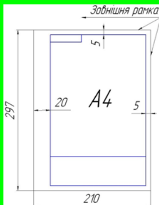
Рис. 10.2 Розміщення основного напису
