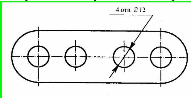
Рис. 2.12 Позначення розмірів декількох однакових елементів
