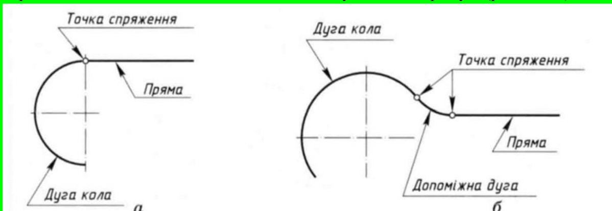
Рис. 13.10 Спряження дуги кола і прямої
