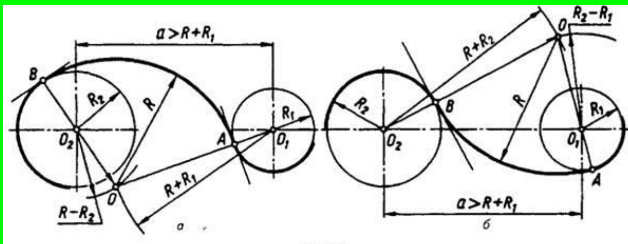
Рис. 13.14 Змішане спряження
