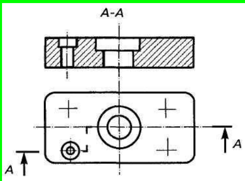
Рис. 15.7 Поздовжній розріз
