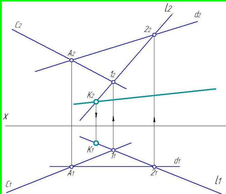
Рис. 4.5 Знаходження точки перетину прямої і площини, заданої двома прямими, що перетинаються
