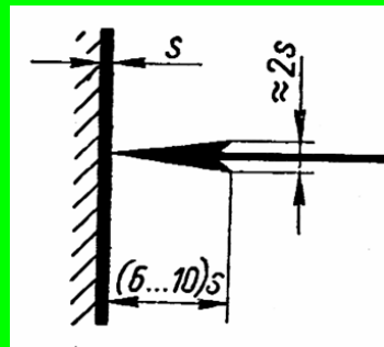
Рис. 12.2 Розмірна стрілка
