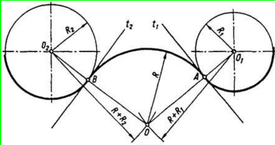
Рис. 13.12 Зовнішнє спряження
