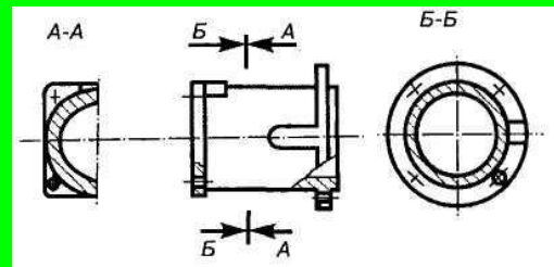
Рис. 15.8 Поперечний розріз
