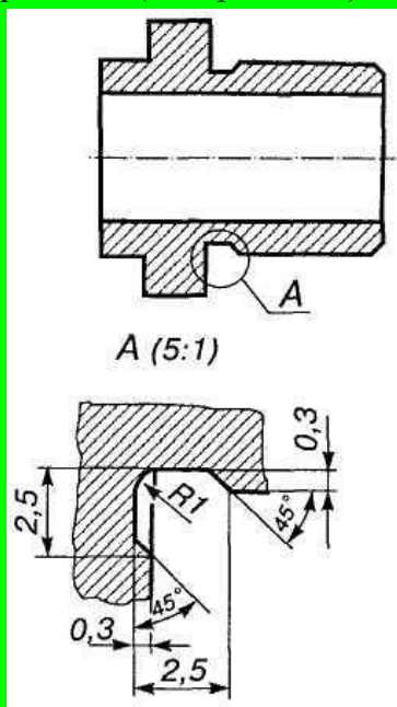
Рис. 7.14 Виносний елемент
