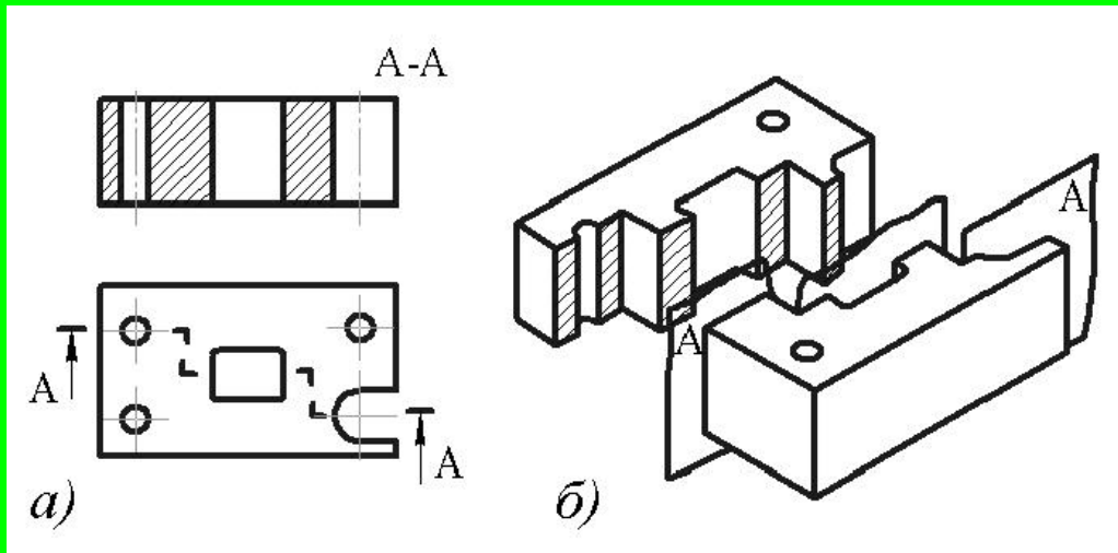
Рис.7.11 Ступінчастий розріз
