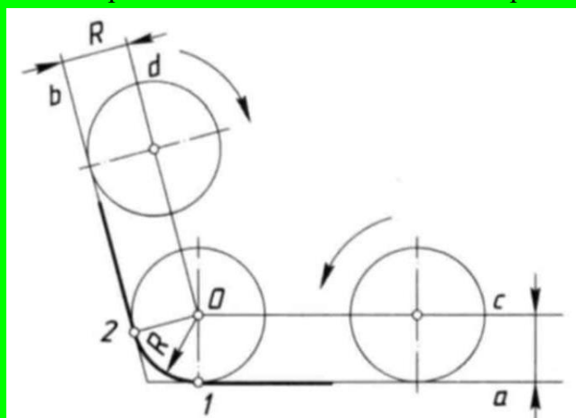
Рисунок 13.7 Принцип побудови спряження
