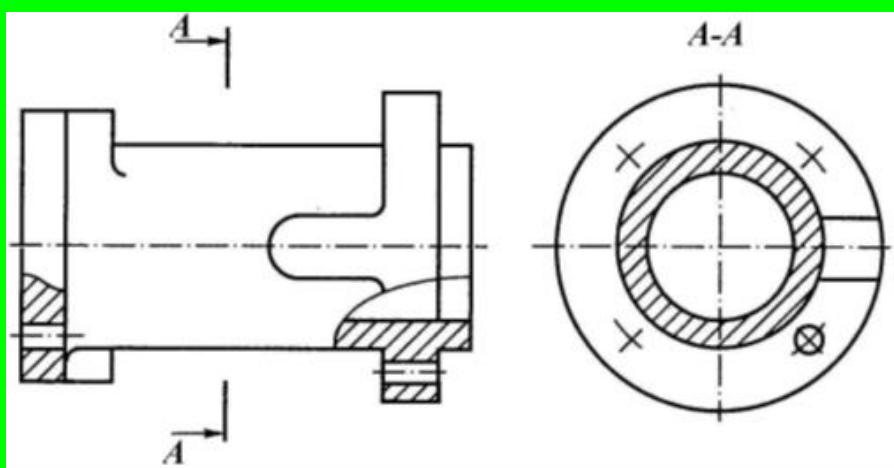
Рисунок 15.9 Позначення розрізу і перерізу
