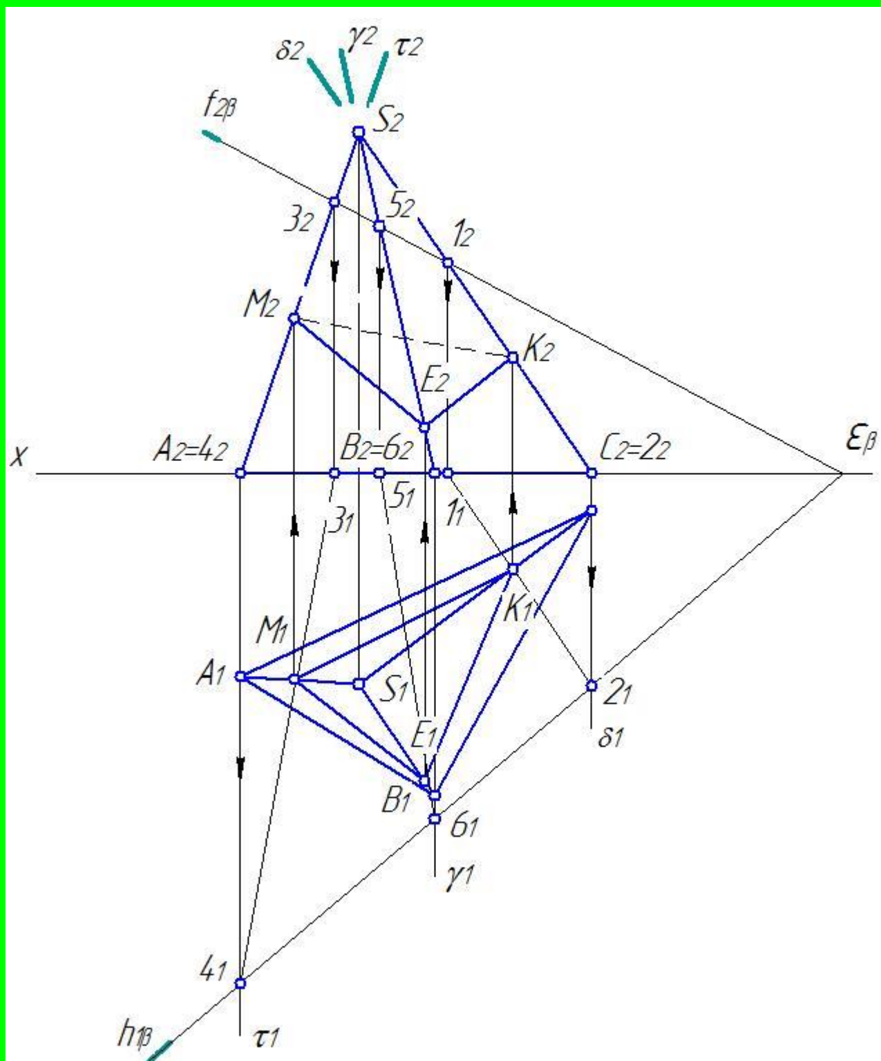
Рис.8.3 Приклад знаходження фігури перерізу піраміди площиною, заданою слідами.
