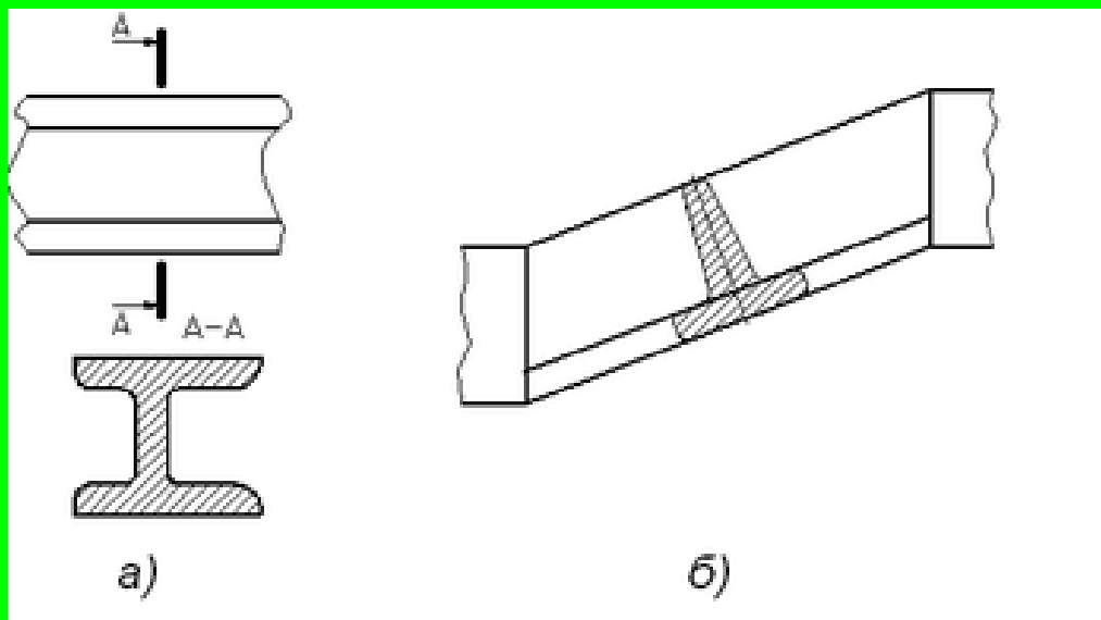
Рис. 7.13 Винесений та накладений переріз
