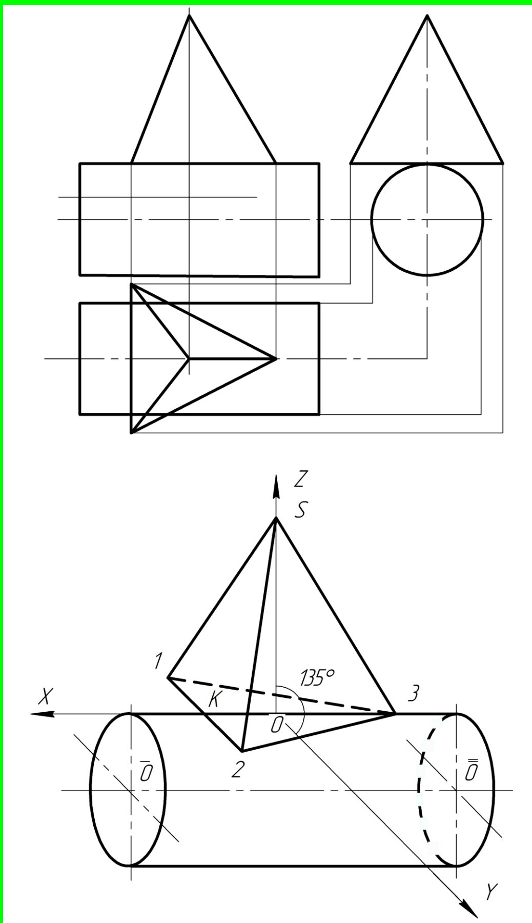
Рис. 3.4 Приклад побудови косокутної фронтальної диметричної проєкції циліндра і піраміди.
