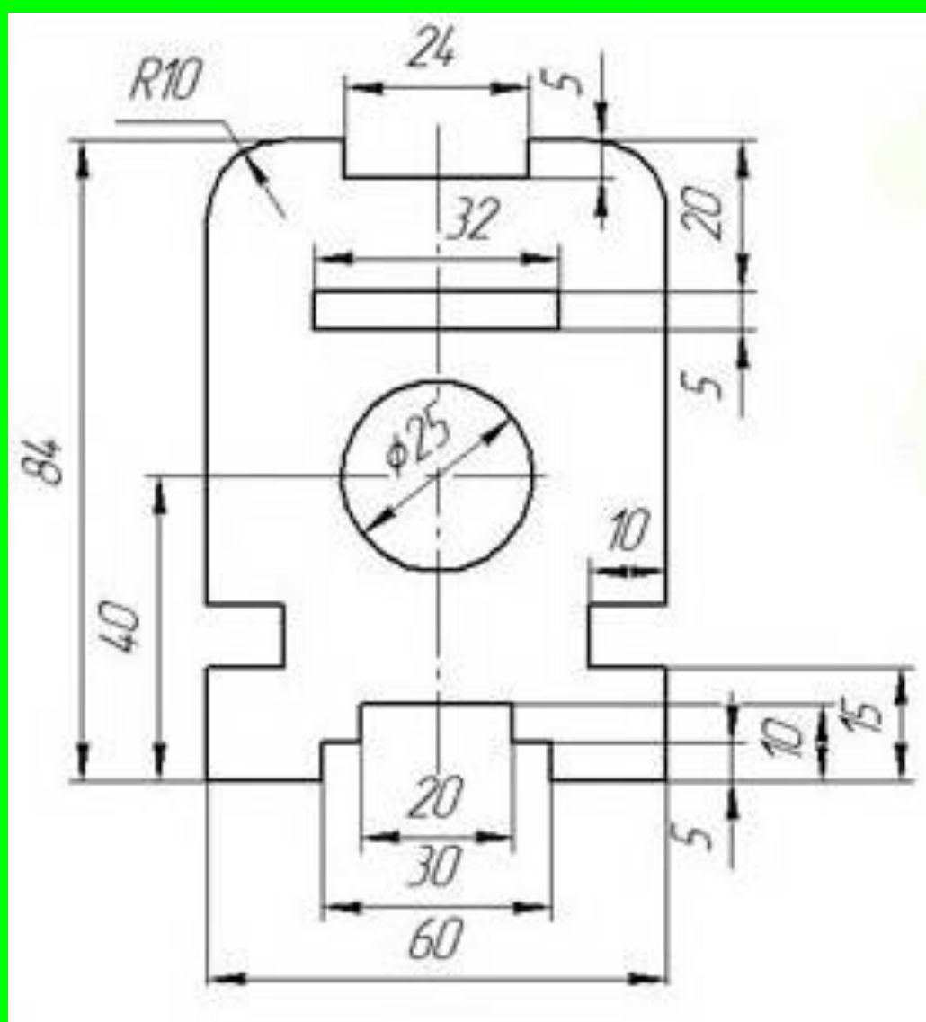
Рисунок 12.17 Зразок виконаної графічної роботи №12
