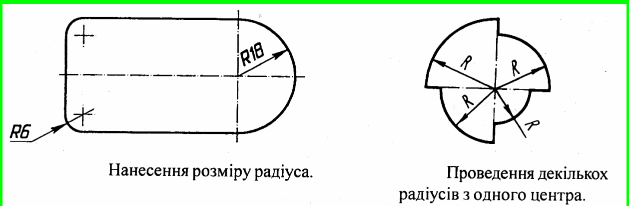
Рис.12.11 Позначення радіусів
