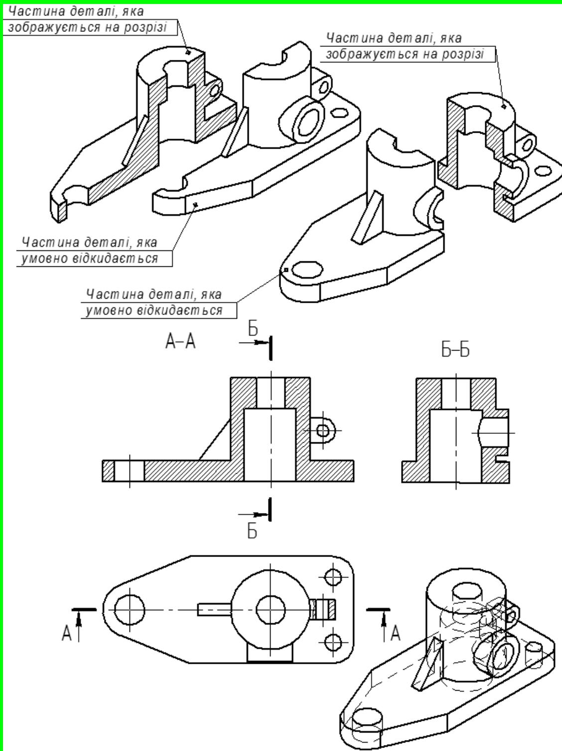
Рис. 15.2 Принцип утворення розрізу
